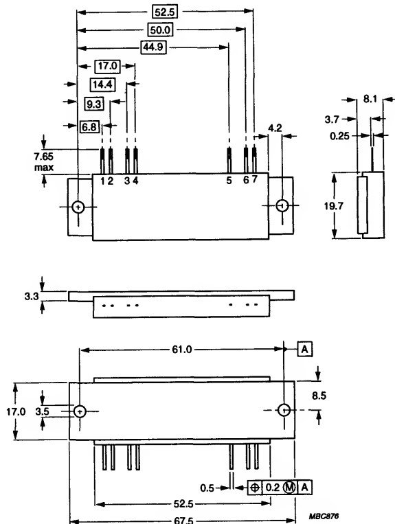
SOT132B
