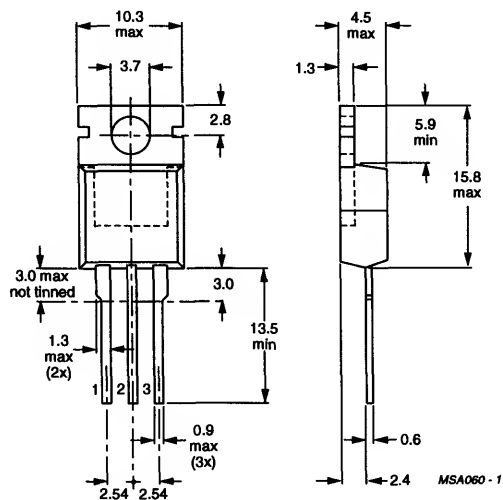
TO220AB
