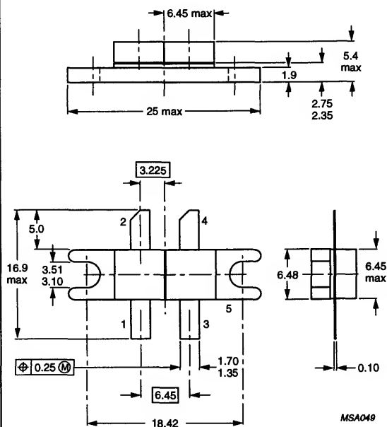
SOT278
