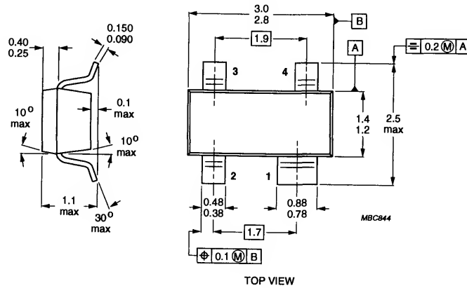
SOT143R
