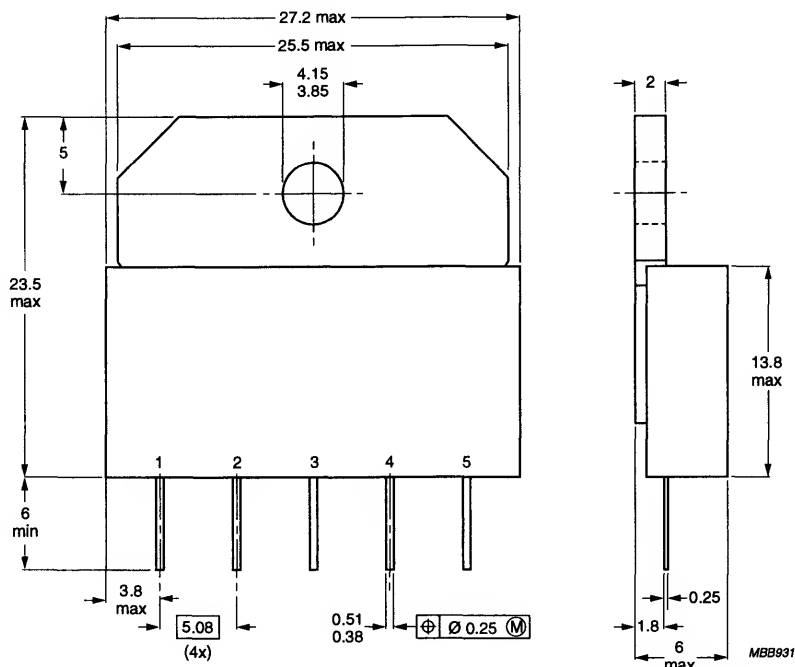
SOT348
