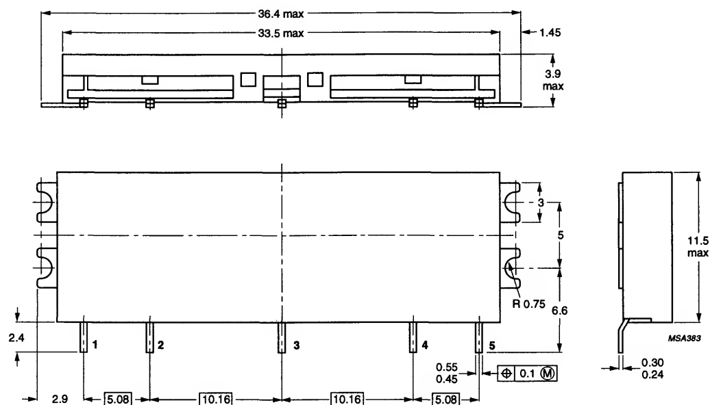
SOT342
