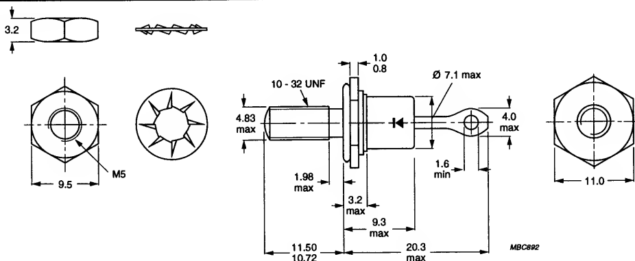
DO-4(1)
