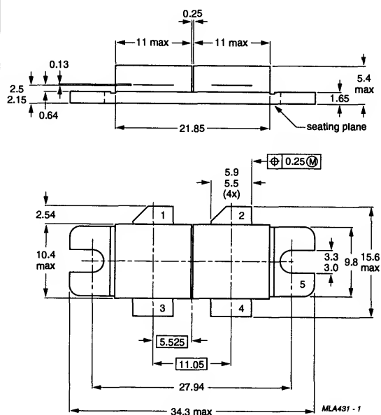
SOT262A2
