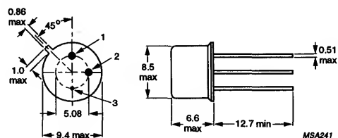
TO-39(b)
