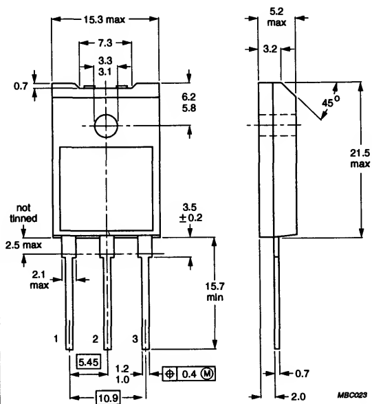
SOT199
