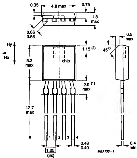
SOT195
