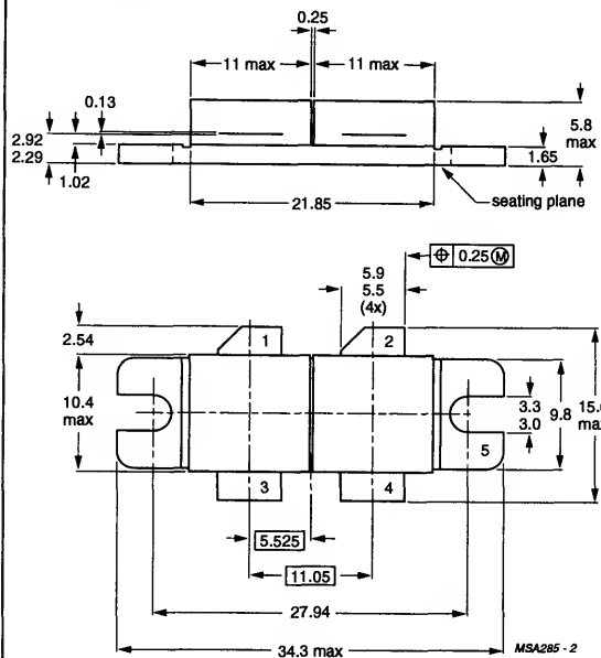
SOT262A1
