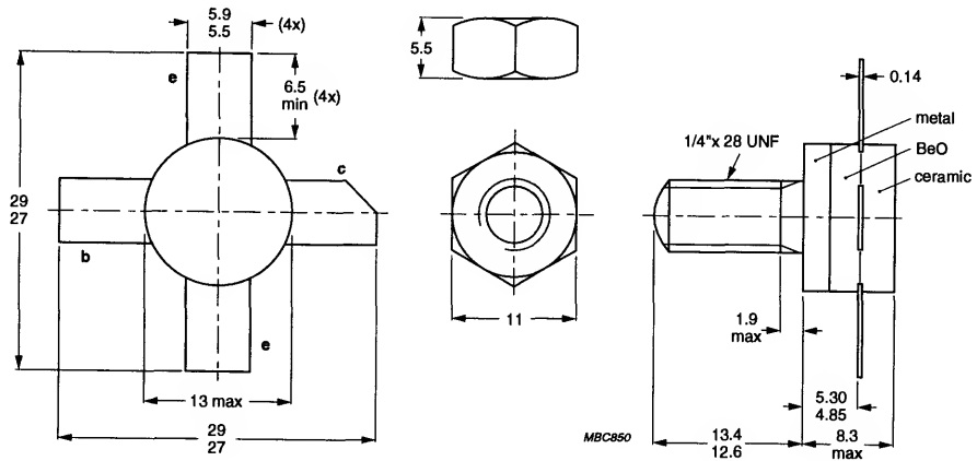
SOT147
