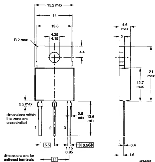
SOT93A
