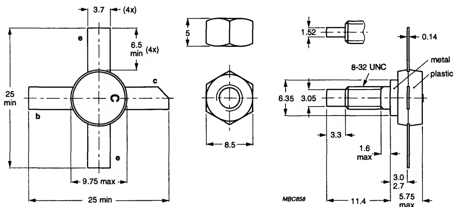
SOT48/2
