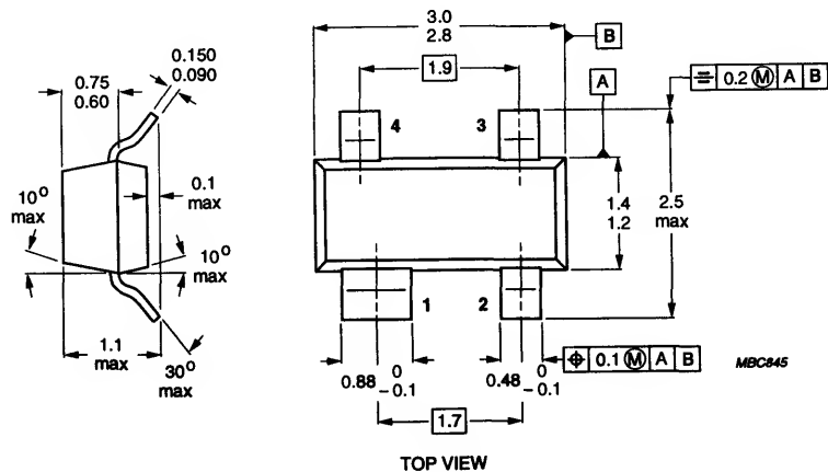
SOT143
