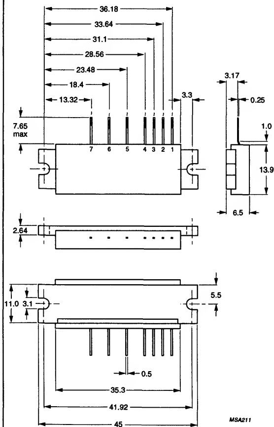
SOT88D
