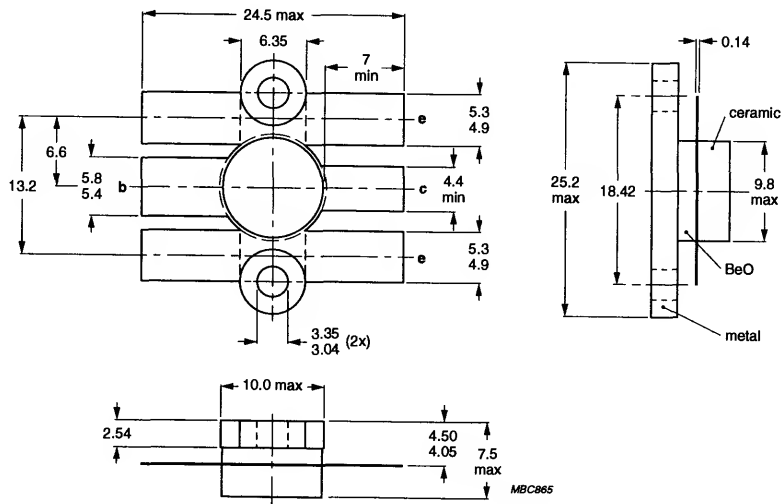
SOT160
