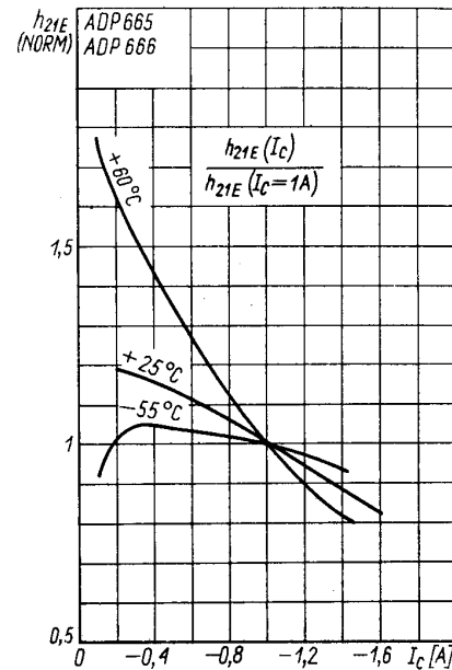
Zależność statycznego współczynnika wzmocnienia prądowego znormalizowanego od prądu kolektora h_{21E(n)} = f(I_C)
