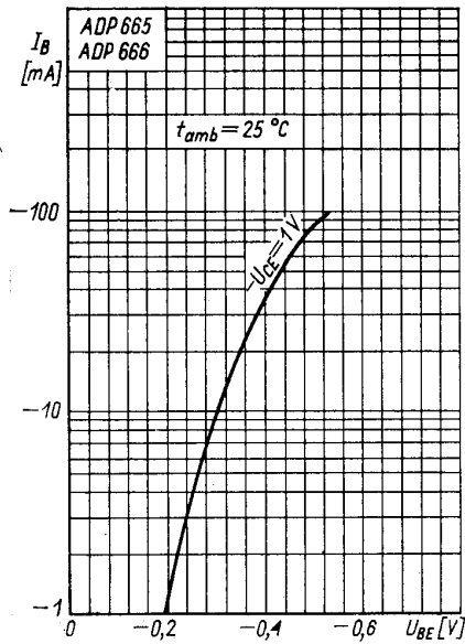
Charakterystyka wejściowa I_B = f(U_{BE}) ; U_{CE} — parametr
