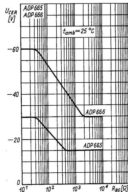
Zależność napięcia kolektor-emiter od rezystancji baza-emiter U_{CER} = f(R_{BE})
