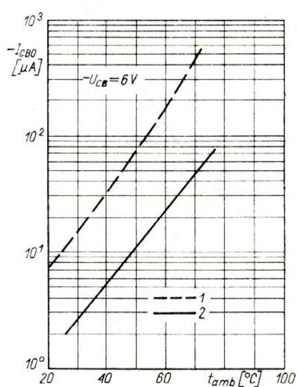
Zależność temperaturowa prądu wstecznego -I_{CBO} = f(t_{amb}) 1 — wartość graniczna, 2 — wartość średnia
