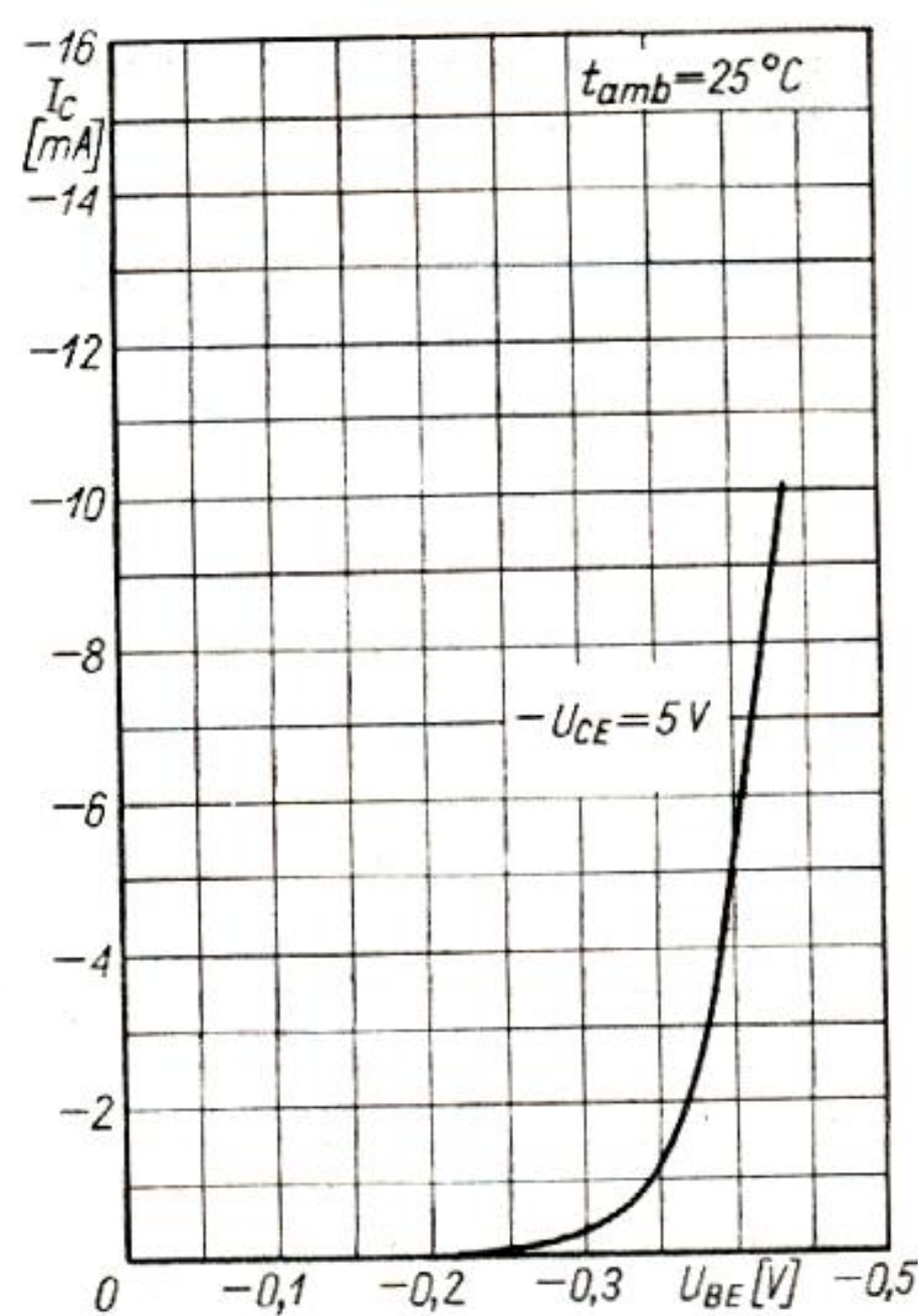
Prąd kolektora I_C = f(U_{BE}) ; -U_{CE} = 5 \text{ V} (Układ wspólnego emitera)
