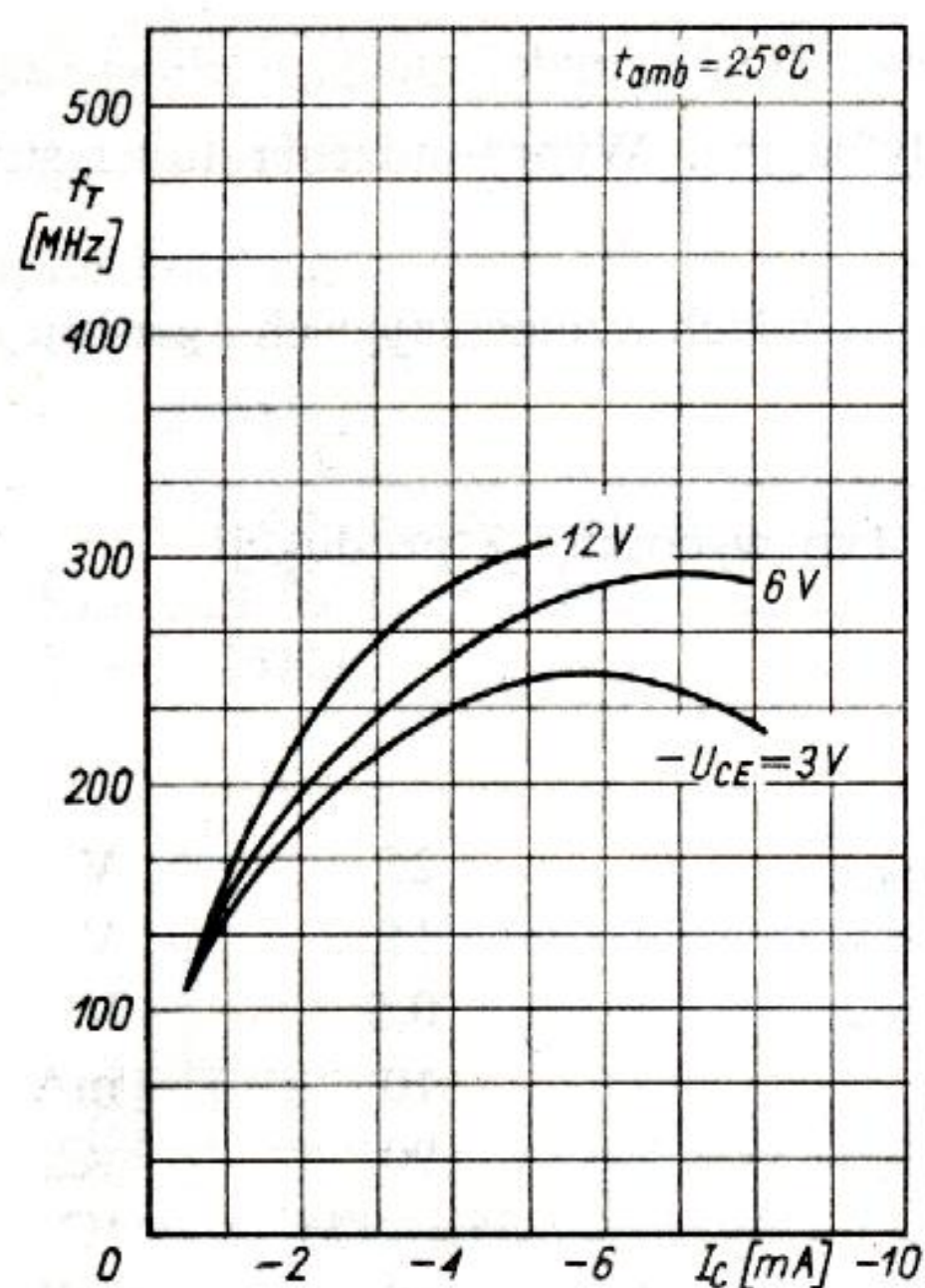
Częstotliwość przenoszenia f_T = f(I_C) ; -U_{CE} = \text{parametr}
