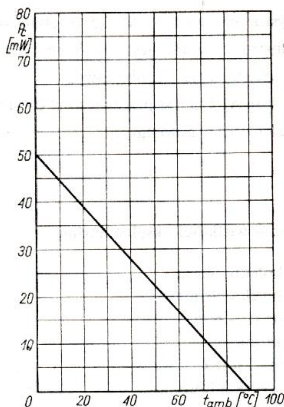
Zależność mocy start kolektora P_c = f(t_{amb})
