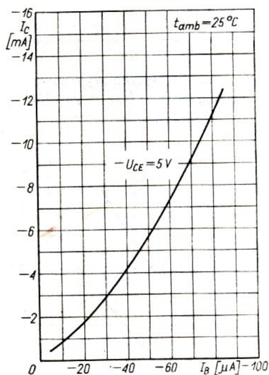
Prąd kolektora I_C = f(I_B) ; -U_{CE} = 5 \text{ V} (Układ wspólnego emitera)
