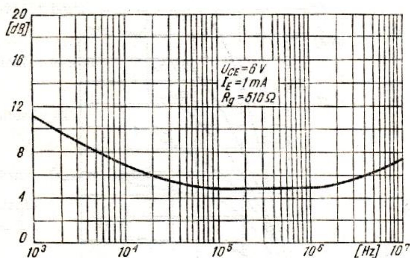
Współczynnik szumów F = f(f)
