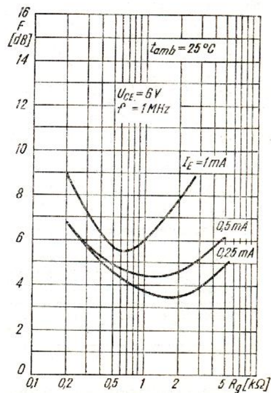
Współczynnik szumów F = f(R_g); I_E = \text{parametr}
