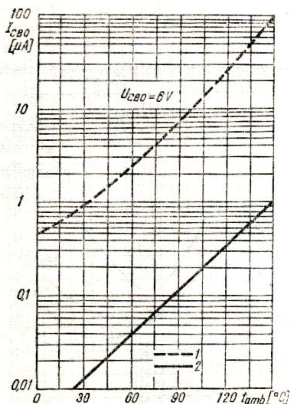
Zależność temperaturowa prądu wstecznego I_{CBO} = f(t_{amb})
