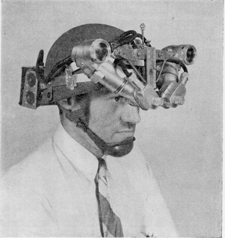
Fig. 12—Type Z Helmet Binocular.
