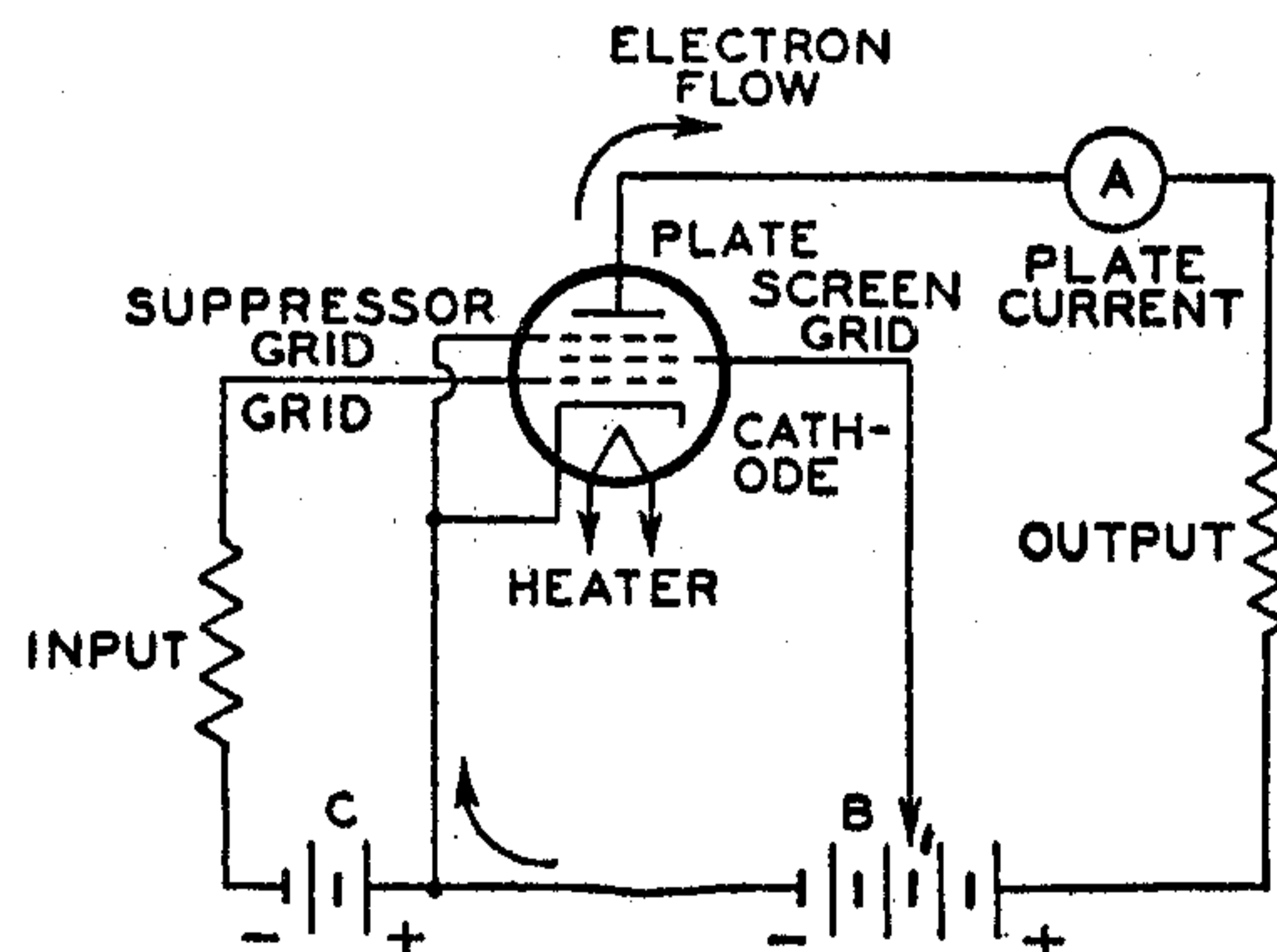
Fig. 8—Basic pentode circuit.
