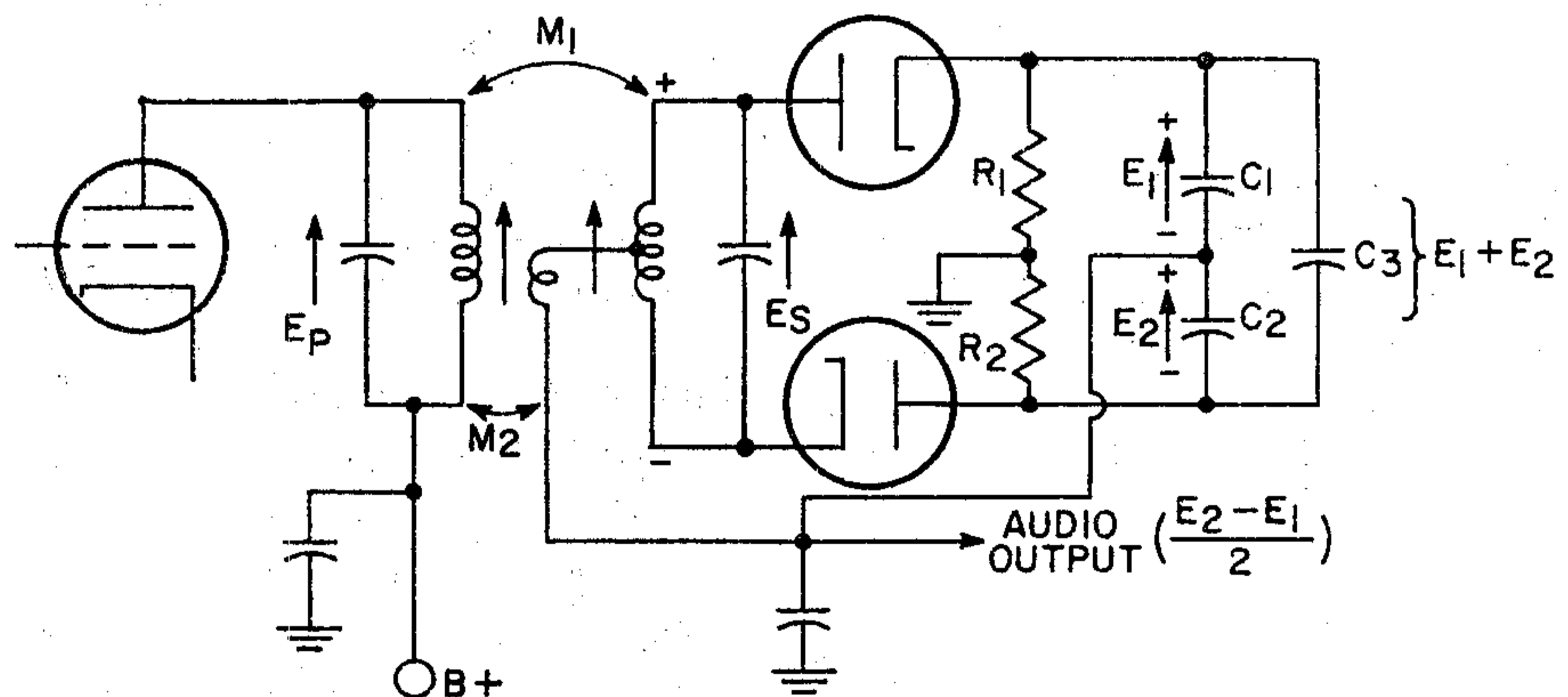
Fig. 33—Radio-detector circuit.
