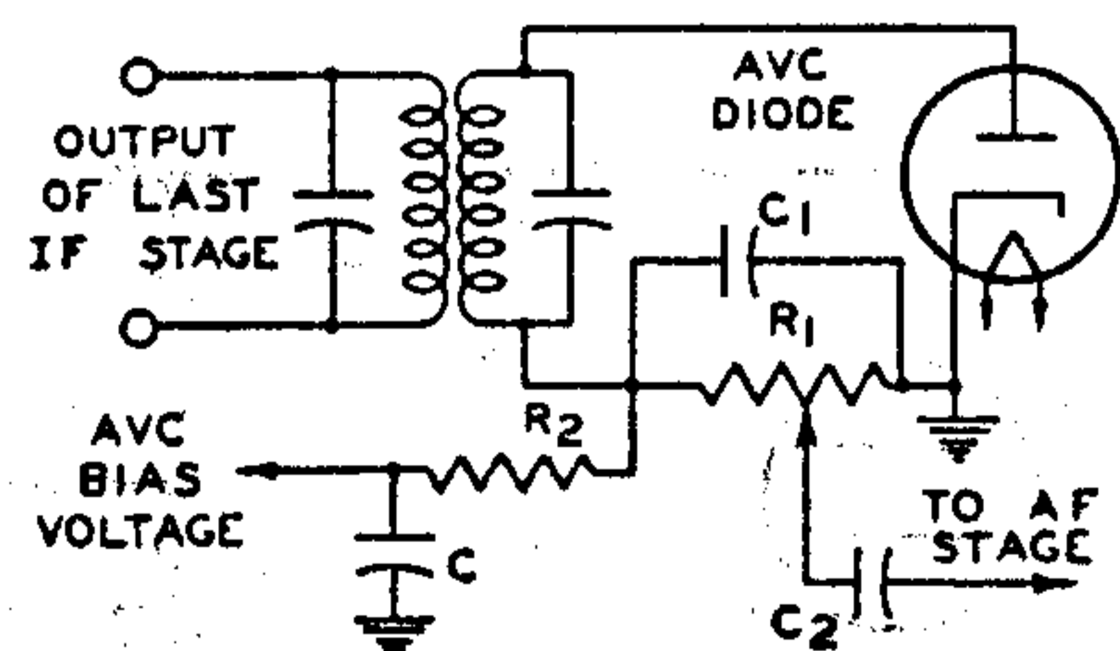
Fig. 61—Automatic-volume-control (avc) circuit.
