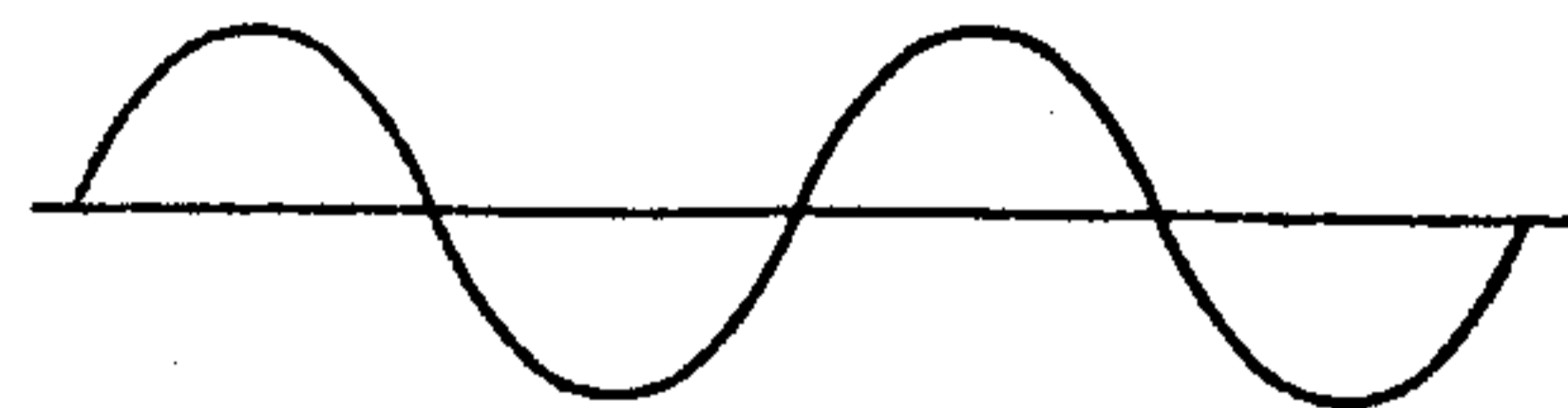
AF MODULATING WAVE
