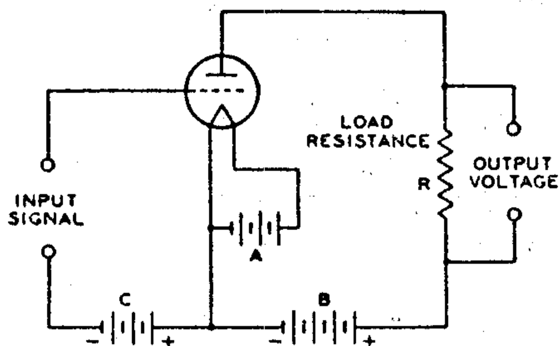
Fig. 35—Triode amplifier circuit.
