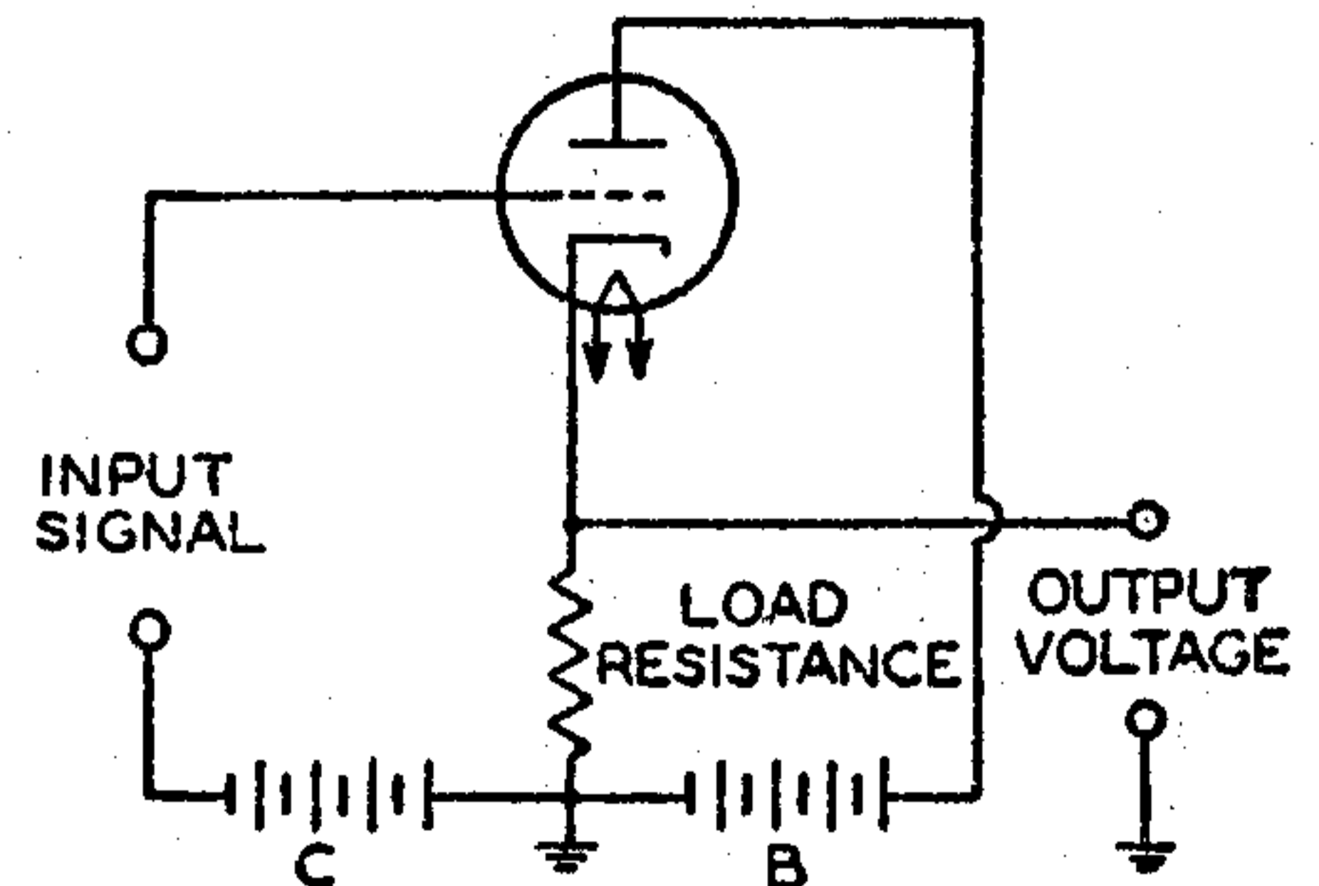
Fig. 51—Cathode-follower circuit.
