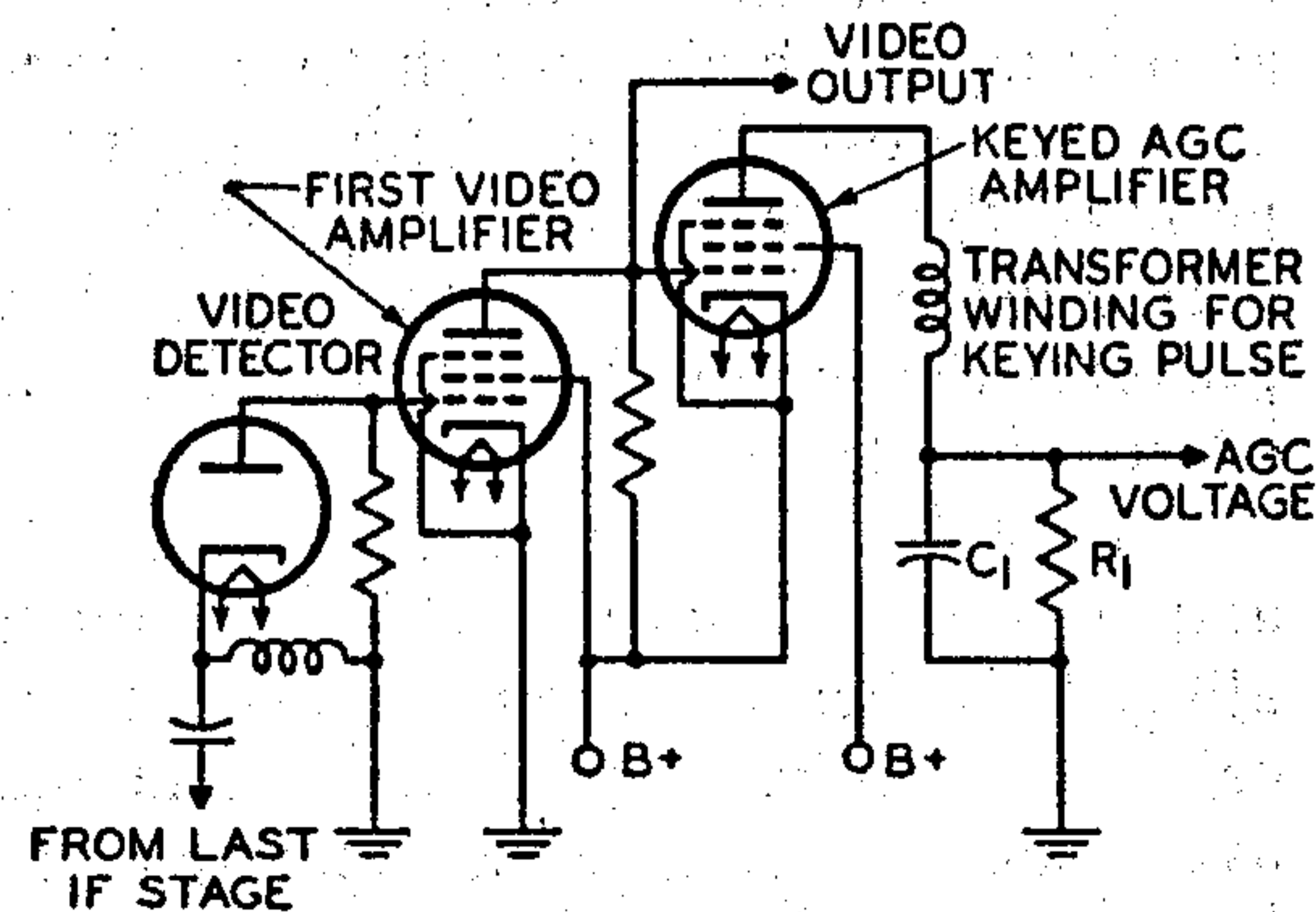
Fig. 64—"Keyed" agc circuit.
