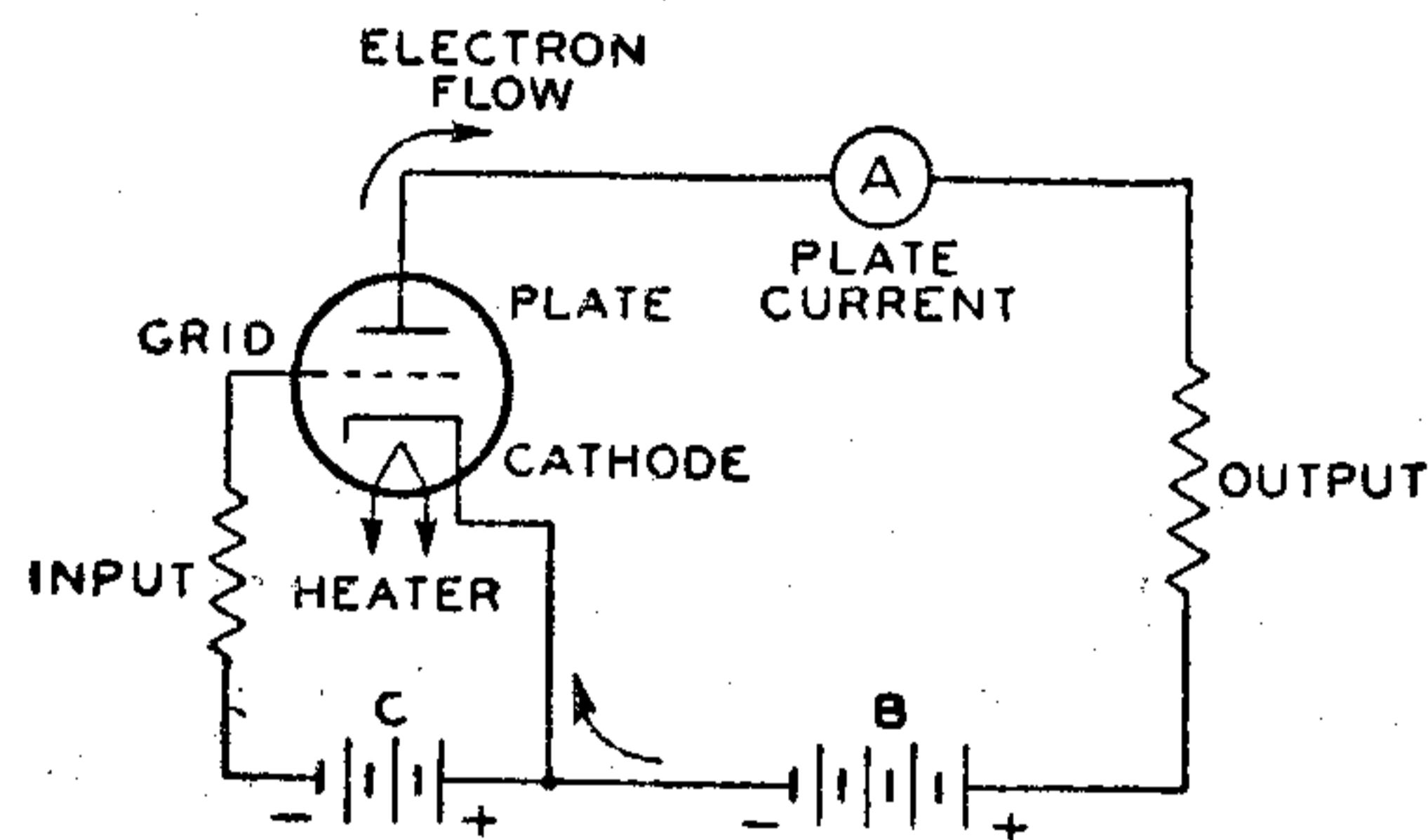
Fig. 6—Basic triode circuit.
