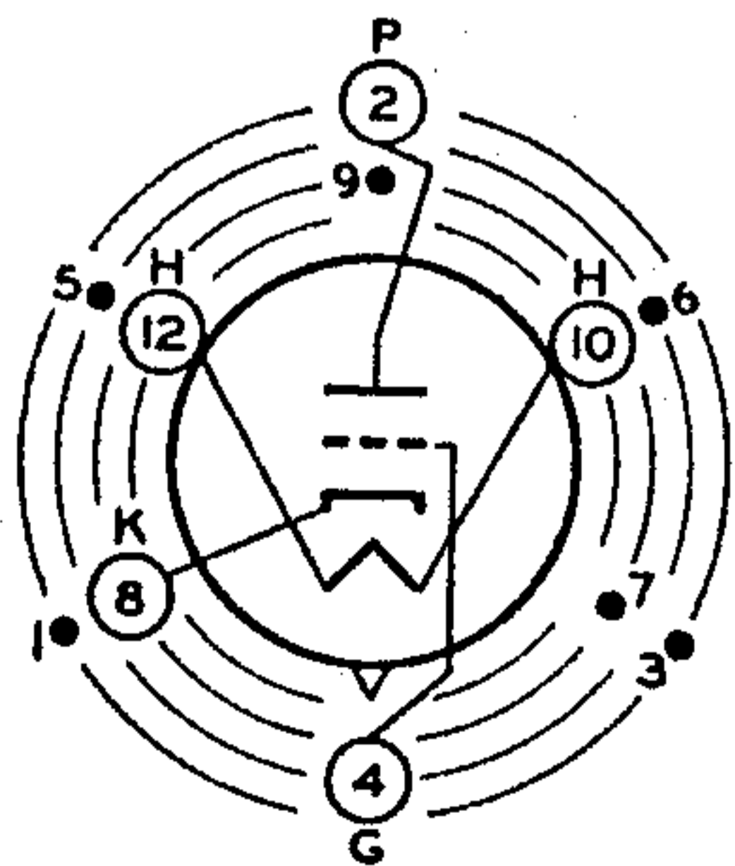
INDEX=LARGE LUG ●=SHORT PIN—IC
