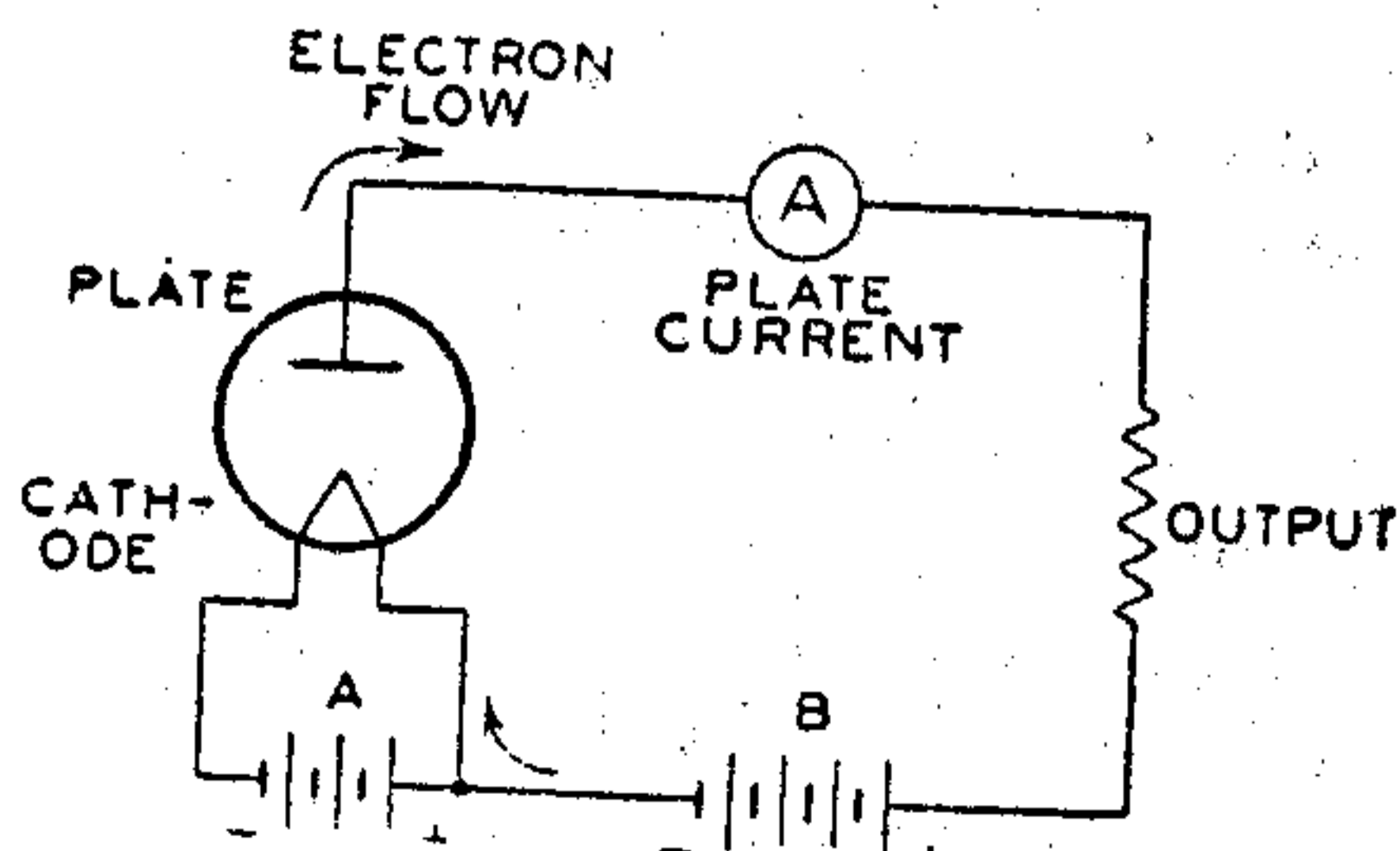
Fig. 3—Basic diode circuit.
