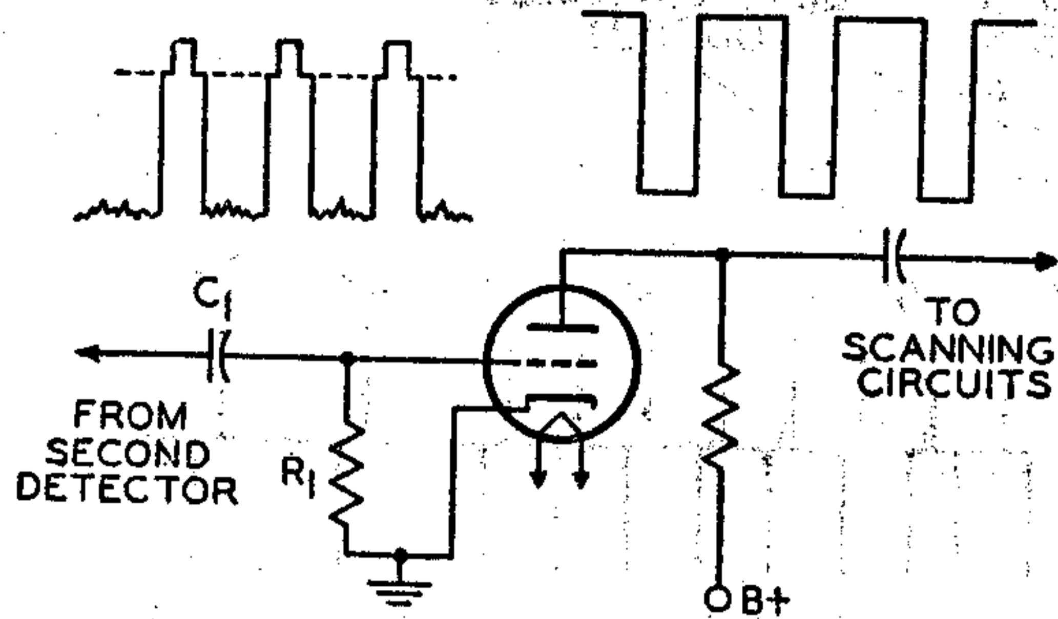
Fig. 80—Sync-separator circuit.
