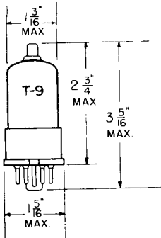
IH5GT/G SKIRTED MINIATURE CAP
