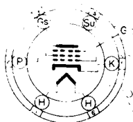
6F BOTTOM VIEW
