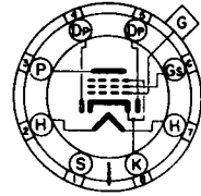
8E BOTTOM VIEW
