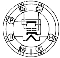
BOTTOM VIEW 6L6G, 6L6GA
