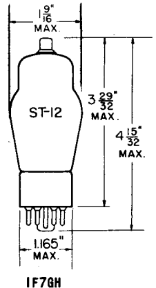
SKIRTED MINIATURE CAP
