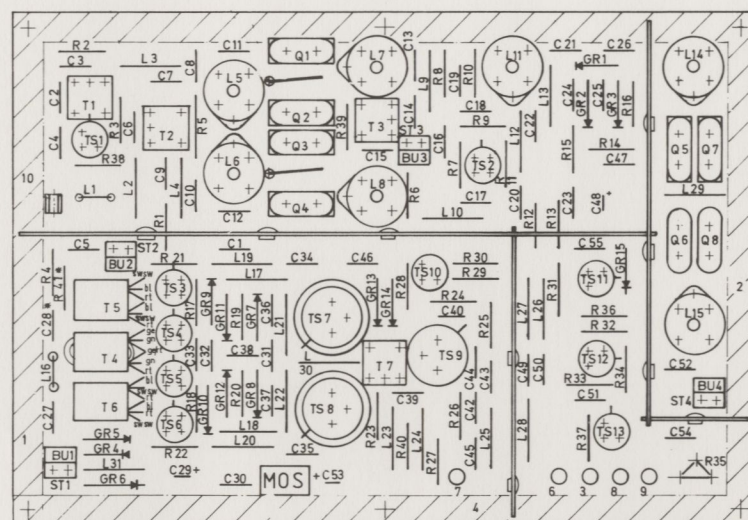
1. Mischer 52.1822.700.00 (07)
