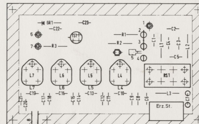
Eingangsfiler 52.1822.100.00 (01)
