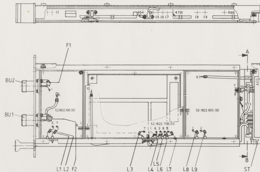
HF-Teil HT 1710/2 52.1822.004.00 (06)
