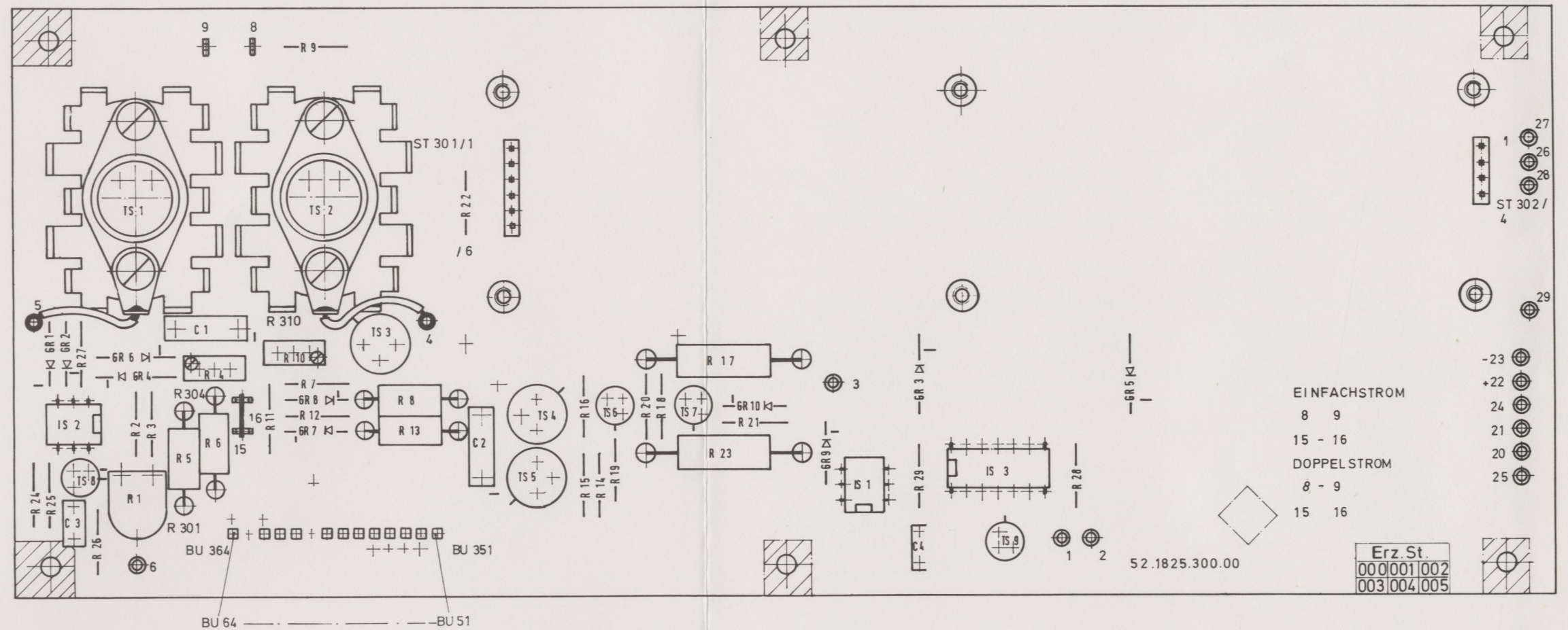
Einfach-/Doppelstromrelais 52.1825.300.00 (01) Beim Aufsuchen in der Schalteilliste zu jeder Schaltteilnummer 300 addieren.
