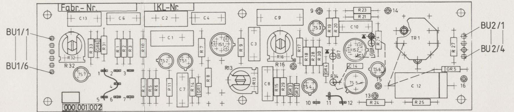
Tontaste 52.1364.280.00 (04) Beim Aufsuchen in der Schalteilliste zu jeder Schaltteilnummer 280 addieren.
