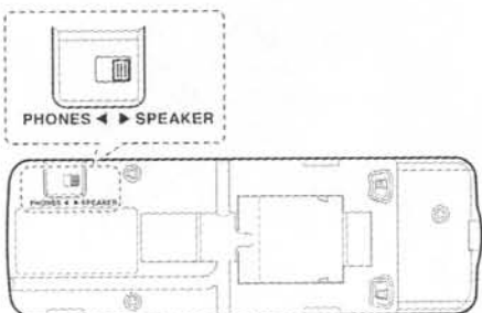
Обратная сторона съёмной передней панели
