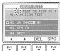
Выбор канала памяти
