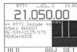
Индикатор RTTY настройки
