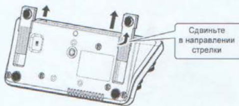
Вид с нижней панели трансивера
