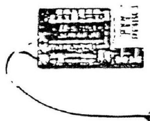
UT-30 CIRCUITO CODIFICATORE DI TONO A 88,5 Hz
