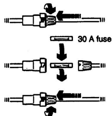
Cavo di alimentazione nella sostituzione dei fusibili
