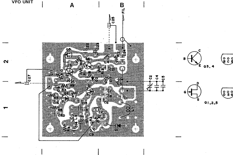
VFO UNIT
