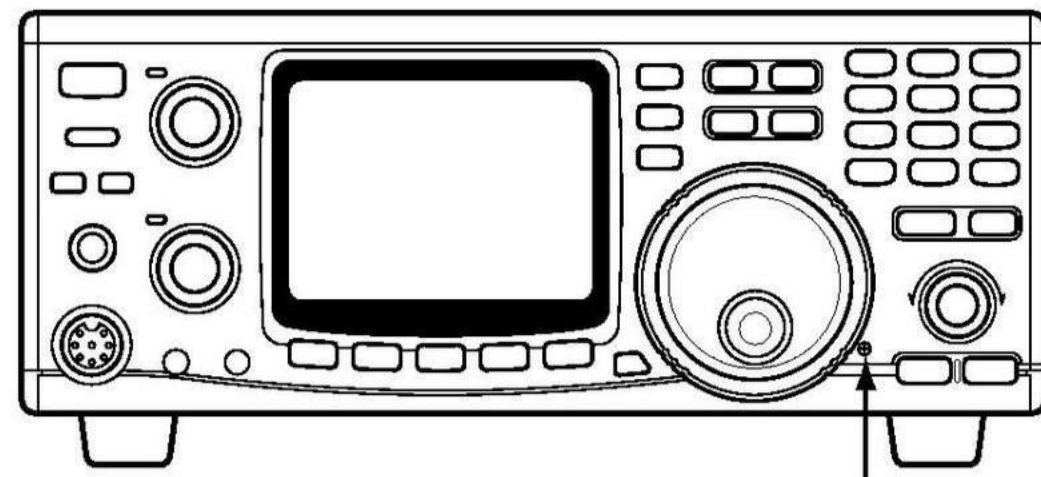
Vite di regolazione
