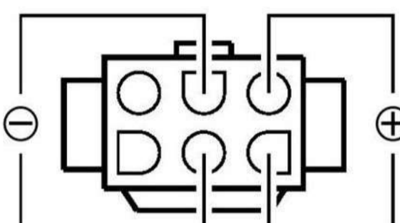
Vista dal lato posteriore
