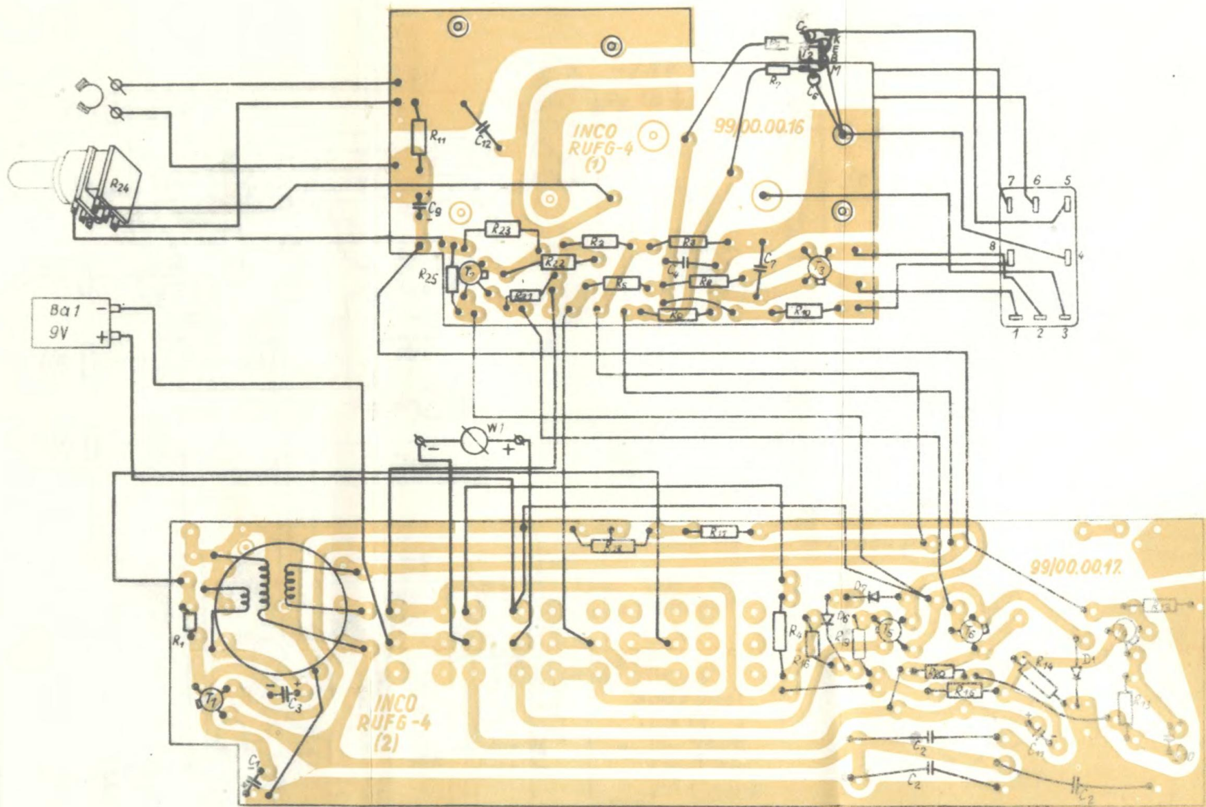
Rys.2 Schemat połączeń poszczególnych podzespołów RUF6-4. Draw.2 Connection diagram of RUF6-4.
