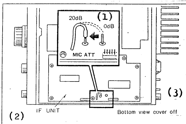
Figura 4.9 - Attenuazione MIC:
