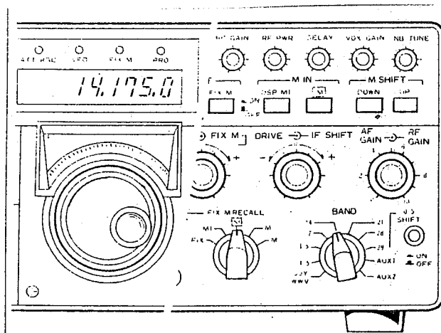
Figura 4.1 - Lettura della frequenza di lavoro.
