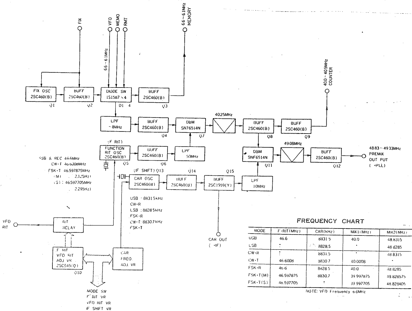
Figura 6.2 - Circuito PRE MIX, del premiscelatore:
