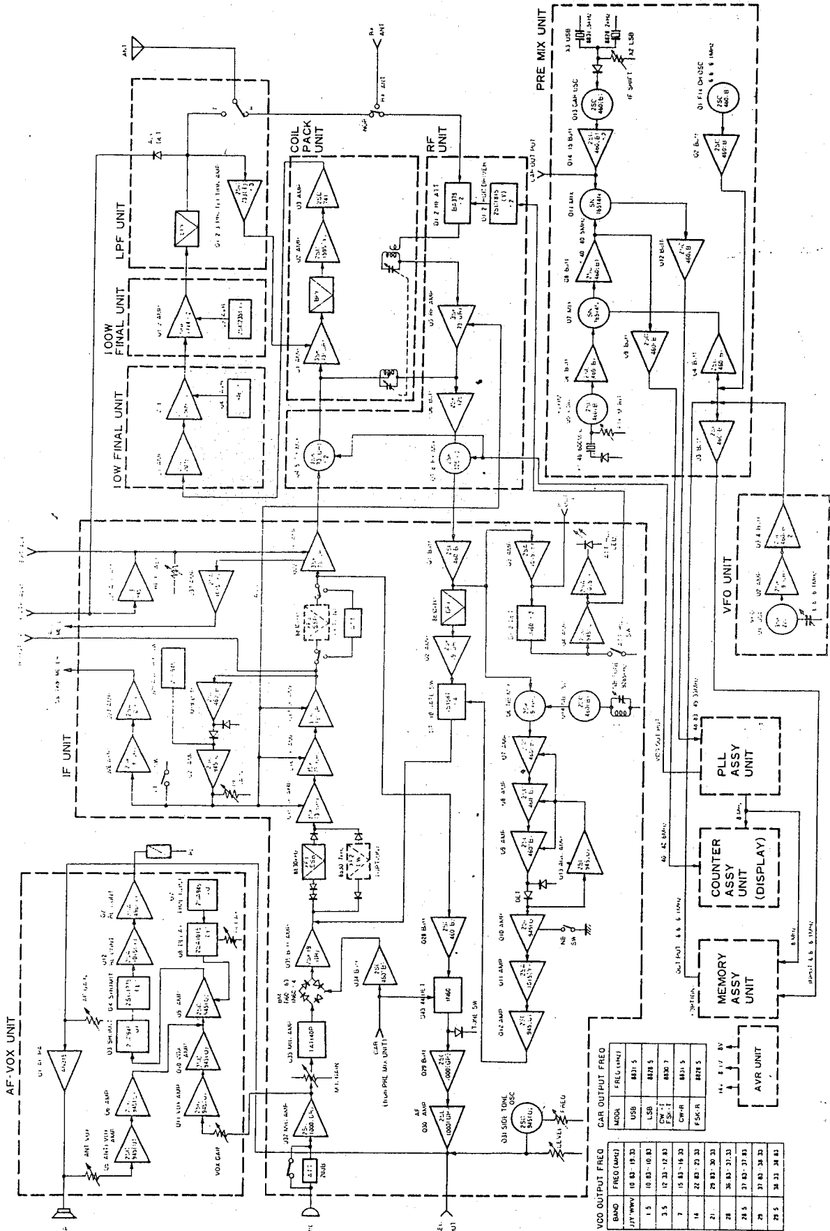
SCHEMA A BLOCCHI
