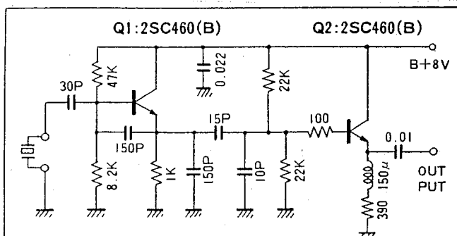
Figura 4.10 - Circuito oscillatore a quarzo:
