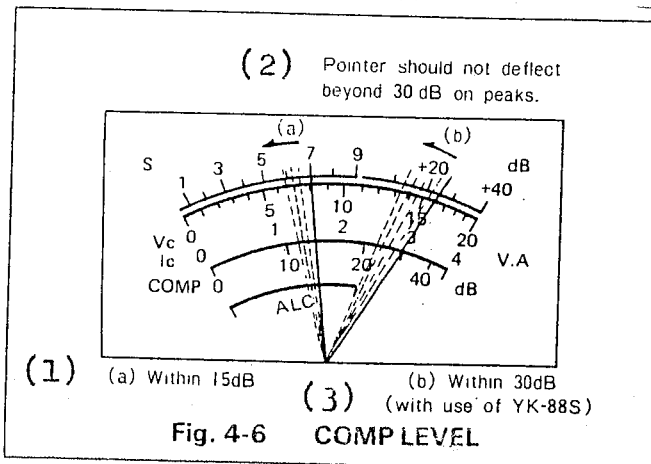
Figura 4.6 - Livello COMP, Compressione.
