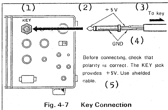
Figura 4.7 - Connessione del tasto:
