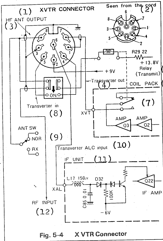
Figura 5.4 - Connettere XVTR : per un Transverter esterno:
