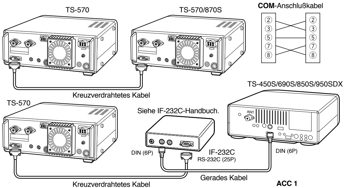
COM-Anschlußkabel
