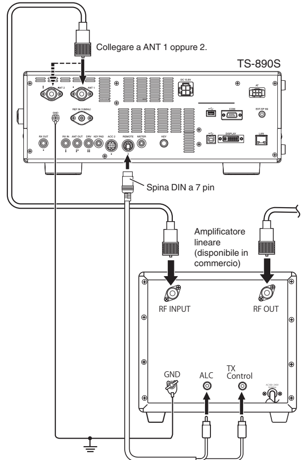
Connettore REMOTE (vista dal pannello posteriore)
