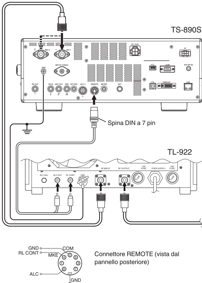
LKY durante Alto attivo/trasmisione: 12 V LKY durante Basso attivo/trasmisione: "L"
