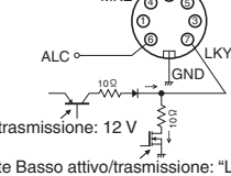
Connettore REMOTE (vista dal pannello posteriore)
