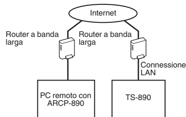
Figura 1: configurazione di base del sistema
