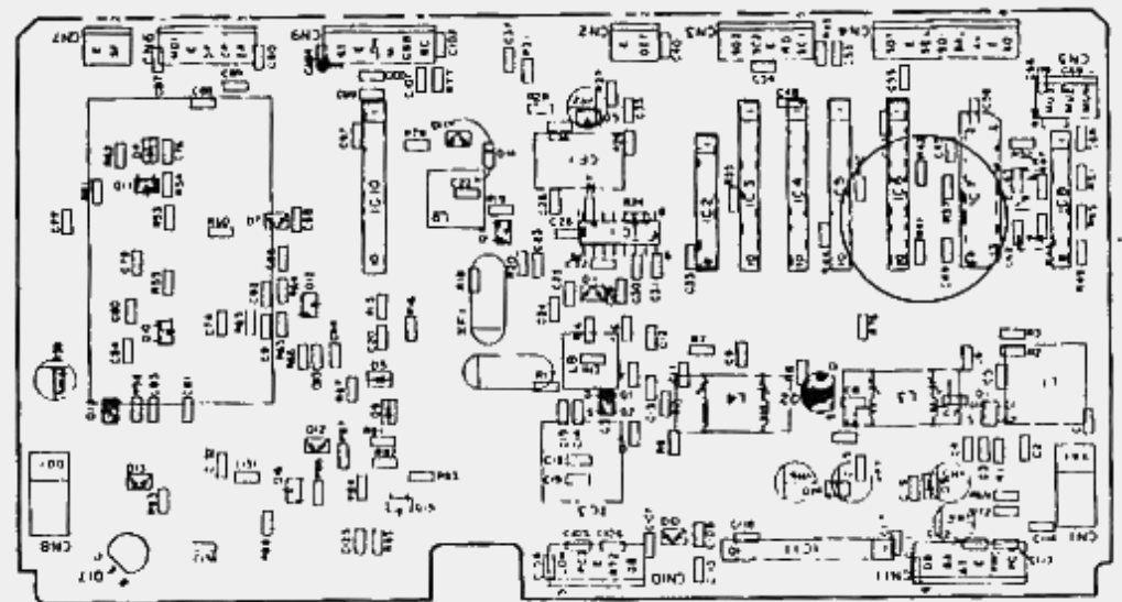
TX-RX (UHF) UNIT
