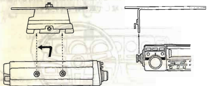
c. セットの取付け
