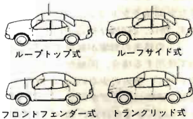
〈アンテナの取付け場所〉
