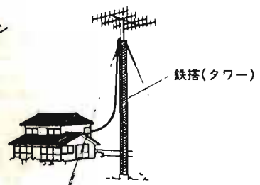
〈本格的なアンテナ〉
