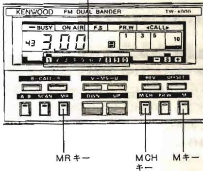
メモリーチャンネル インジケーター
