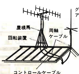
〈八木アンテナをスタック(積重ね)した例〉
