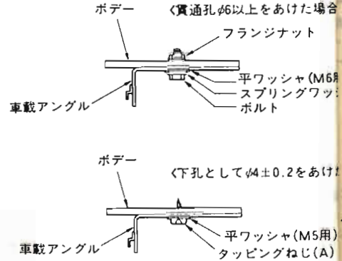
b. 車載アングル取付け
