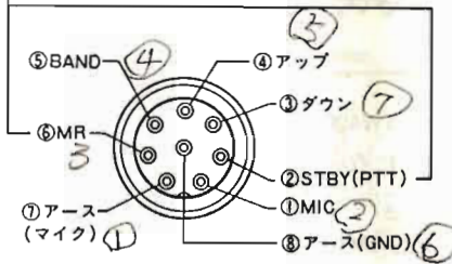
〈パネル面から見た図〉
