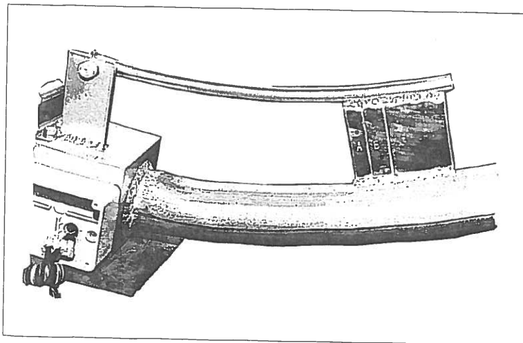
Particolare del gamma match della Midi.
