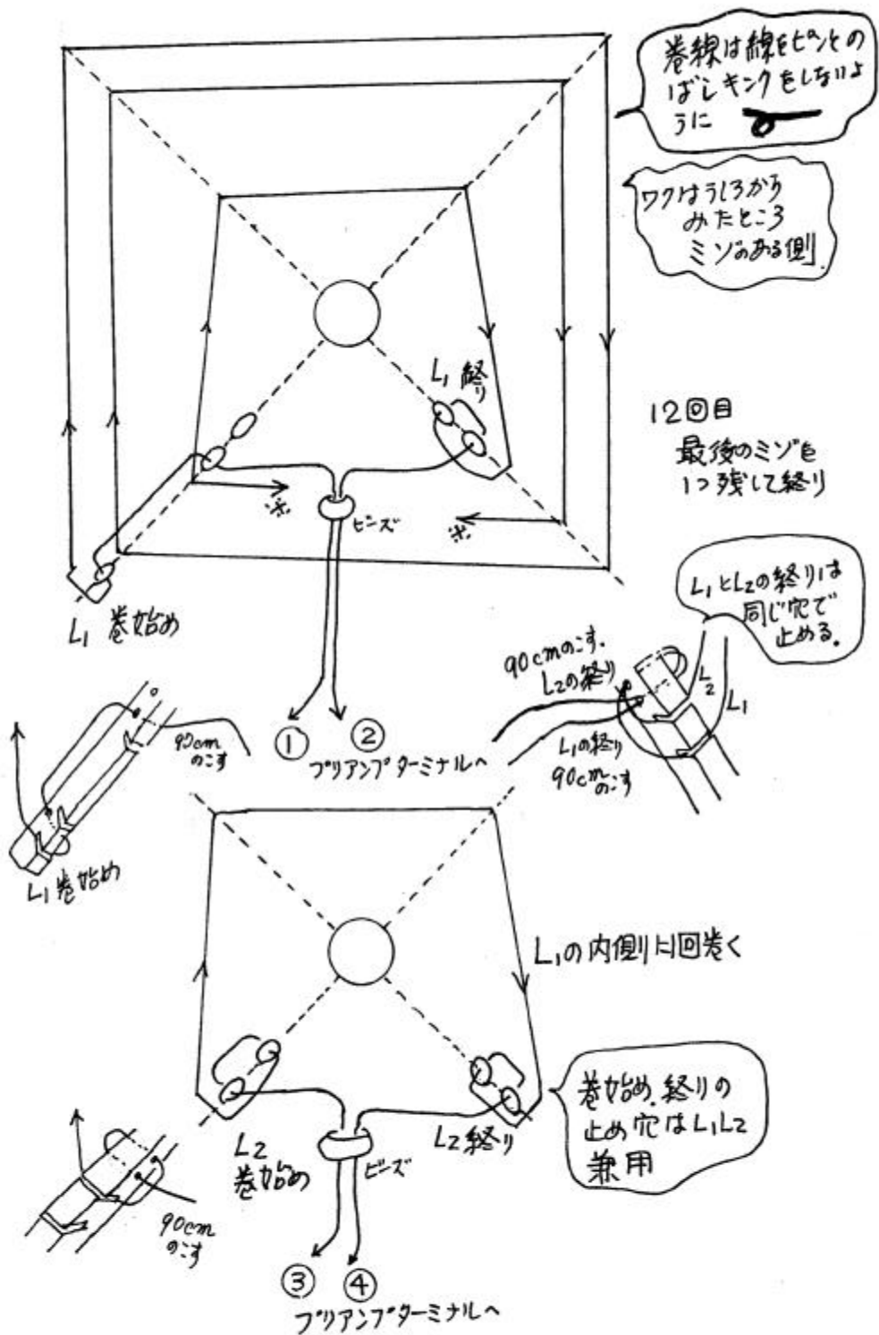
第8図 ループアンテナの巻きかた
