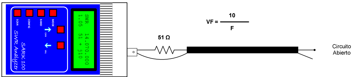
Ilustración 12, Determinando el factor de velocidad de una línea
