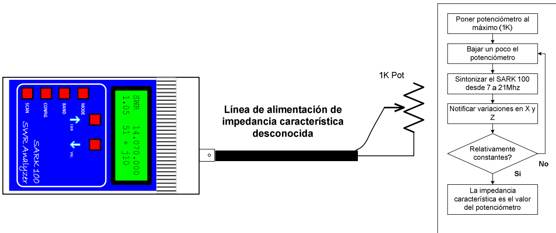
Ilustración 11, Determinar la impedancia característica de una línea
