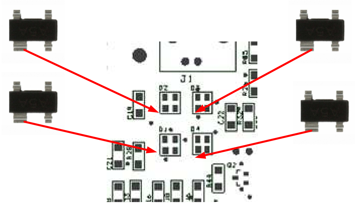
Ilustración 2, Orientación de D1..D4
