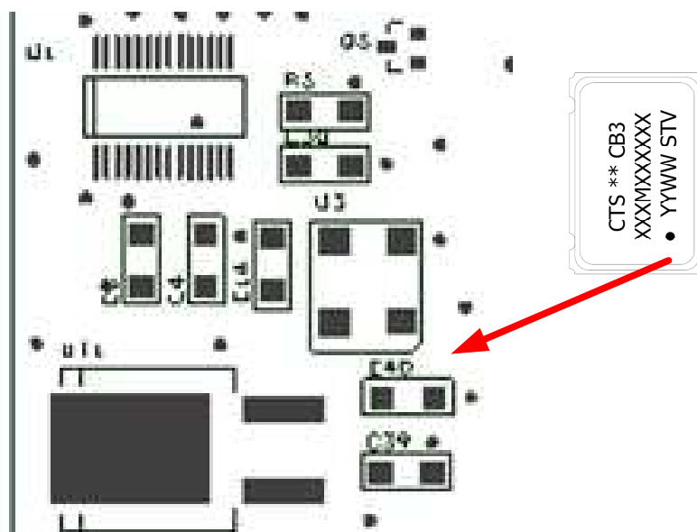
Ilustración 3, Orientación de U3
