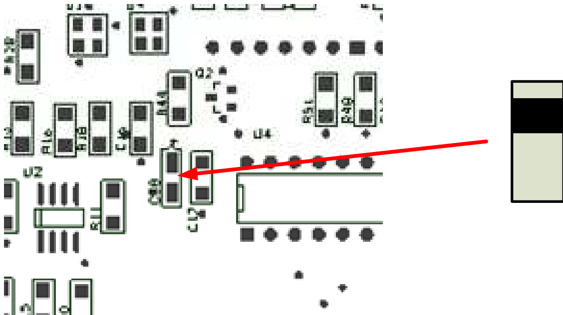
Ilustración 4, Orientación de D5, D6, D7
