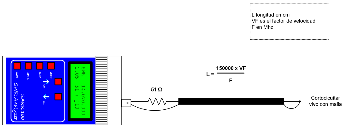
Ilustración 8, Ajuste de acopladores de antena
