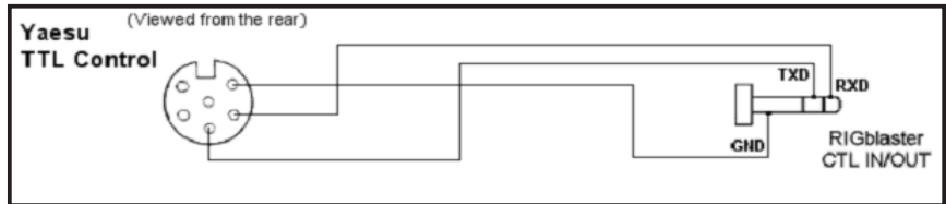
Yaesu 6 pin DIN CAT control cable wiring
