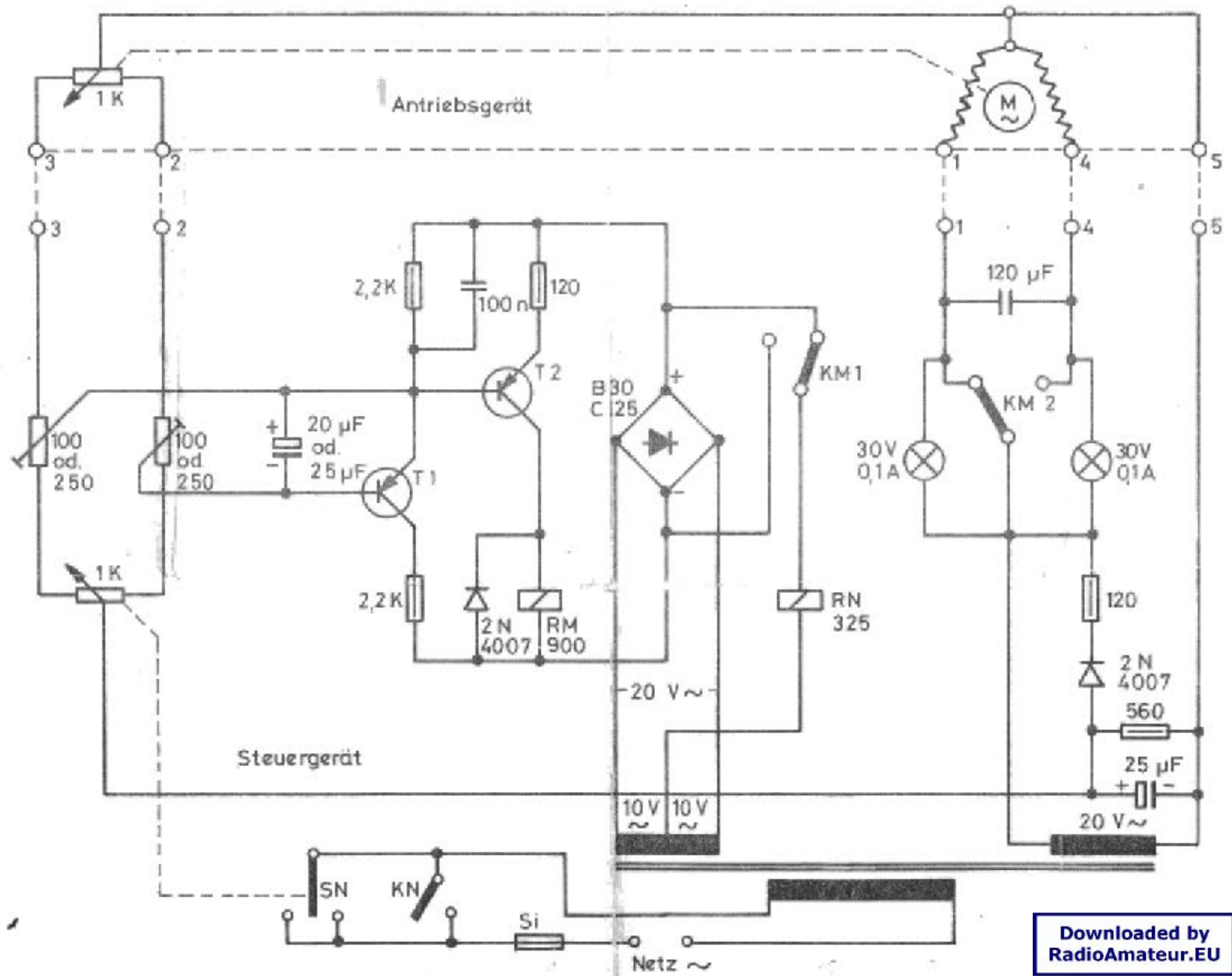
Schaltbild, Antennen-Rotor Typ 2010/220; 2040/220
