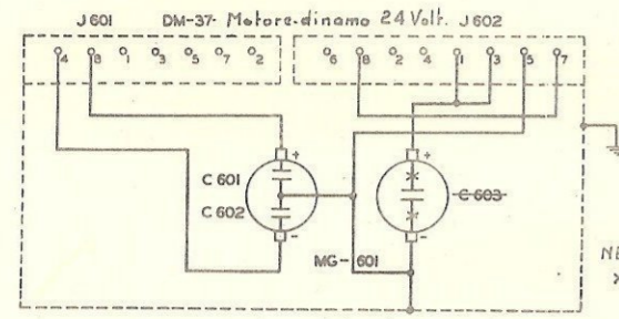
R-508; R-528-AN/VRC-5. Circuito elettrico Trasmittitore BC-604
