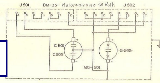
Jack microfono magnetico
