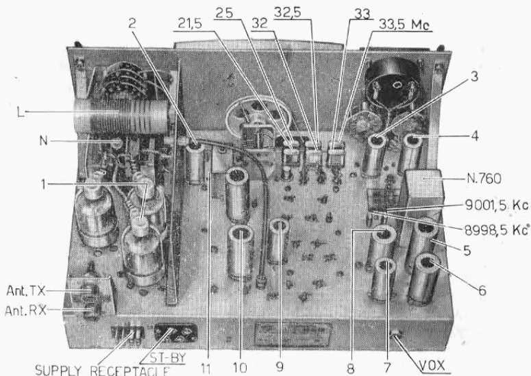
Vista posteriore del trasmettitore G 4/228
