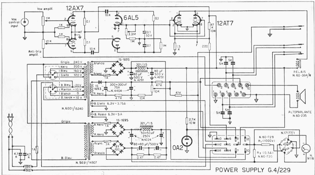
Schema elettrico alimentatore 4/229
