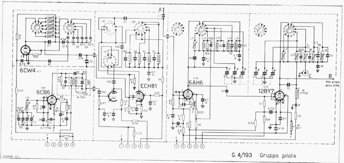
Schema elettrico gruppo pilota 4/193
