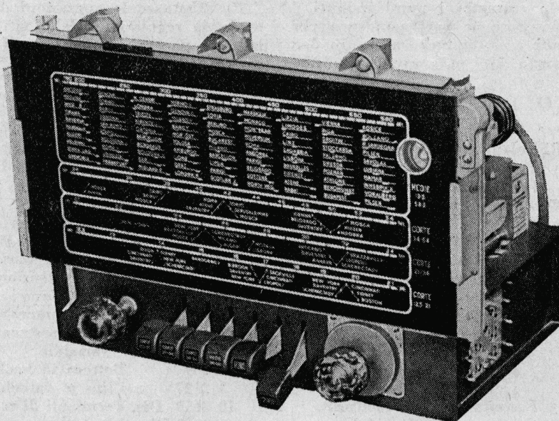
Fig. 1 - Radiorecettore G-77R.
