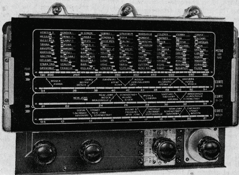
Fig. 1 - Radiorecettore Super G-503.
