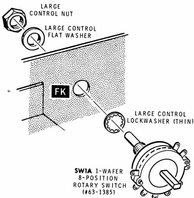
Detail 15-4E
