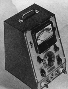
RCA-Rider Voltohmmyst—20A
