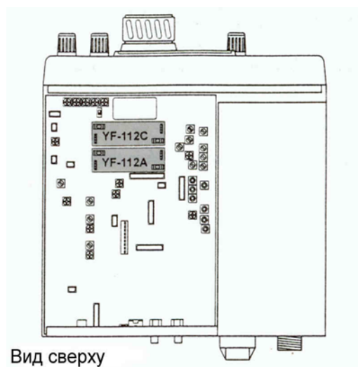
Рисунок 2. Установка кварцевых фильтров.
