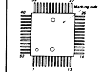
μPD7508G-779-00
