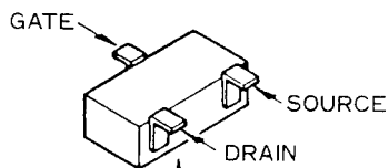
2SK160 (K6) (Q3019)
