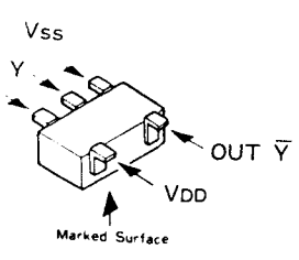
TC4S584F(CA) (Q6052, Q6061)
