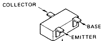
2SC2712GR (LG) (Q3002, Q3003, Q3012, Q3013, Q3035, Q3036, Q3054, Q3055) FA1A4P (L34) (Q3018, Q3021, Q3022, Q3026, Q3033, Q3037, Q3038, Q3046, Q3058, Q3060, Q3063, Q3068, Q3070, Q3071, Q3078, Q3079) FA1F4N (L35) (Q3067) FN1A4P (M34) (Q3047, Q3059, Q3061, Q3084)
