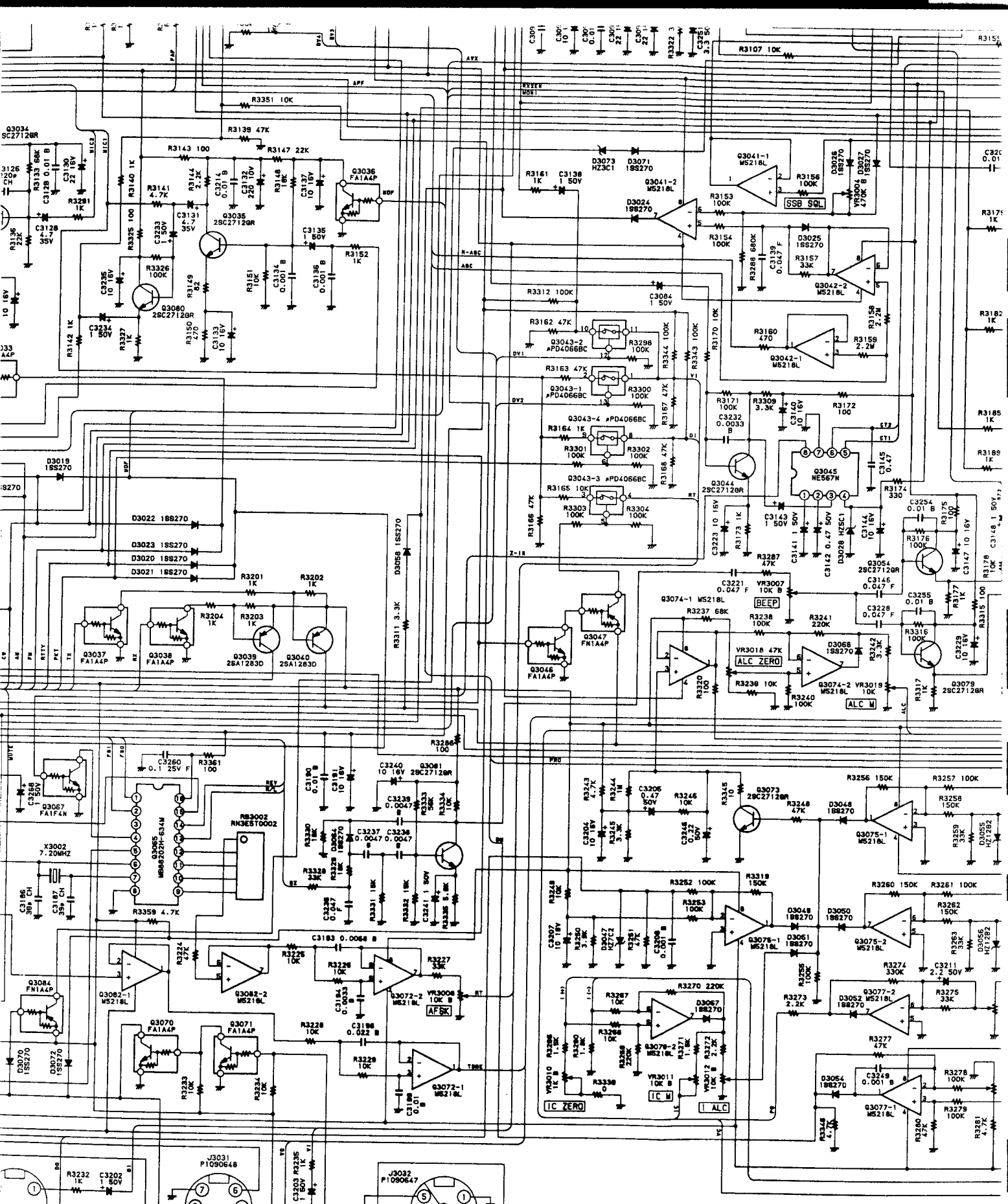
AF UNIT F3061101C
