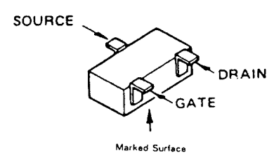
2SK302GR(TG) (Q6069) 2SK302Y(TY) (Q6056, Q6070)
