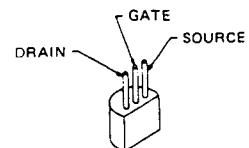
2SK125 (Q1009, Q1010, Q1015, Q1016, Q1017, Q1018, Q1021, Q1036, Q1037)
