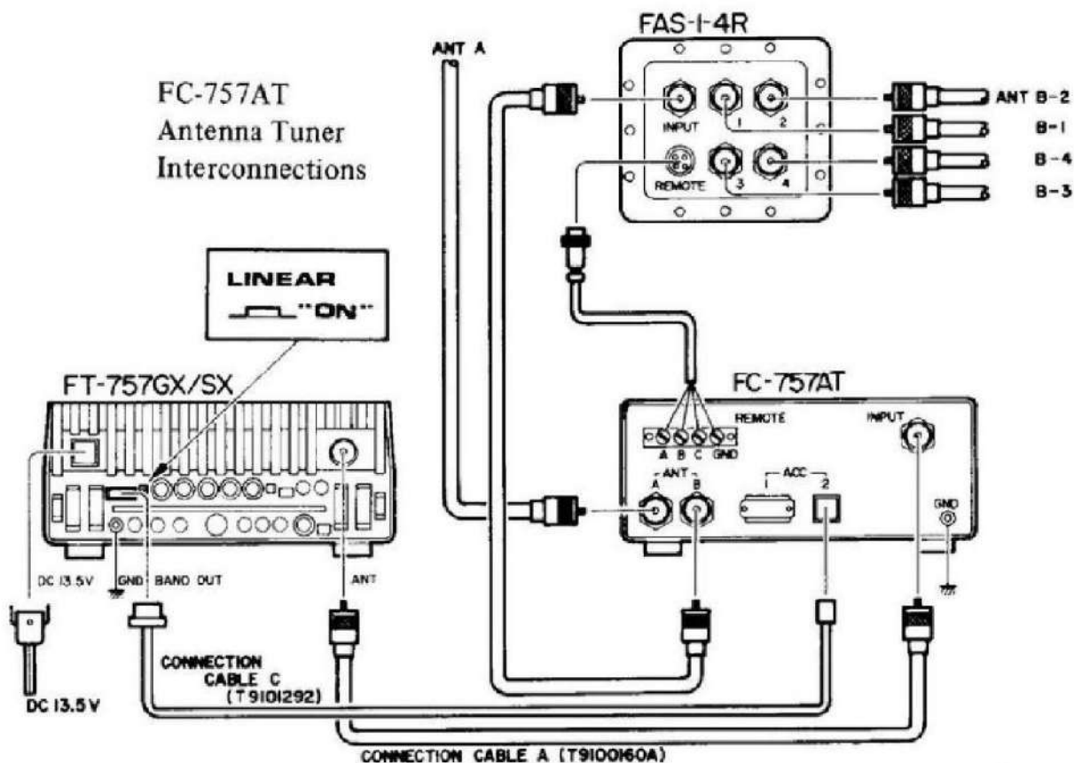
VITE REGOLATRICE DEL FRENO
