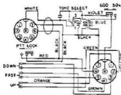
MD-1 BB
