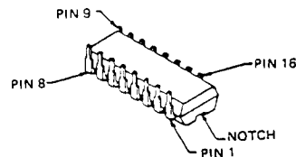
MC14049UBCP (Q1060)
