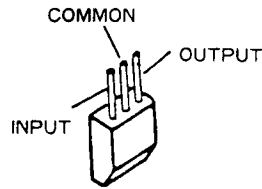
μPC78L05 (Q7010)
