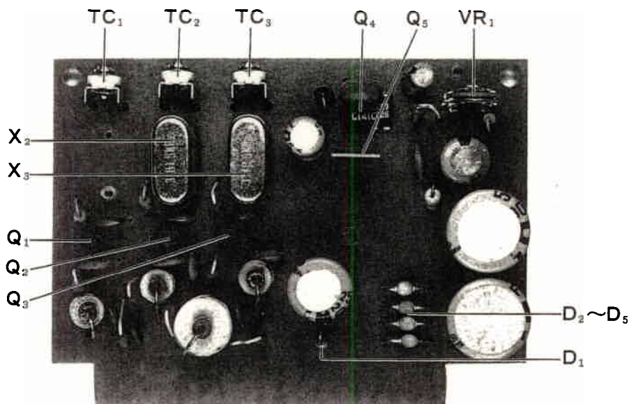
Fig. 17 REG-BFO UNIT
