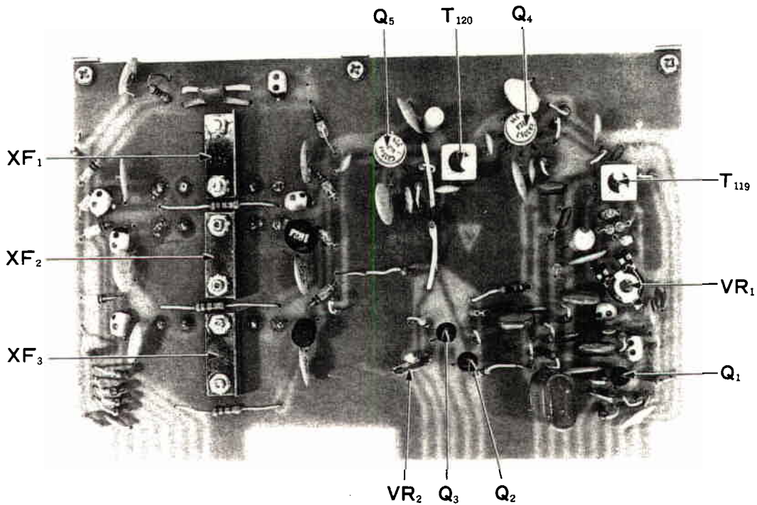
Fig. 15 IF UNIT
