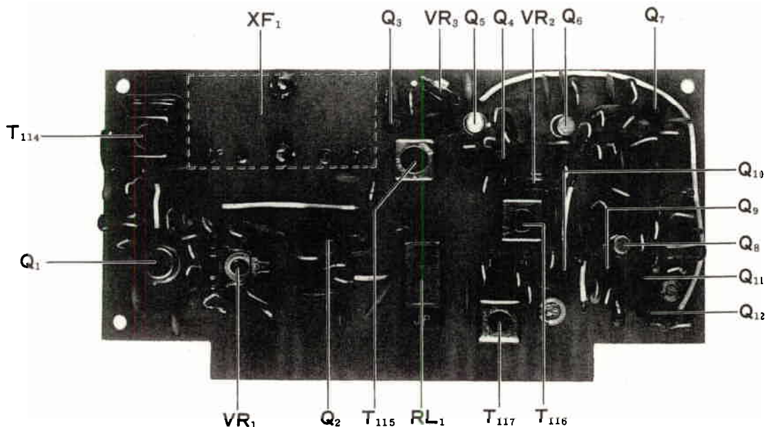
Fig. 14 NB-MIX UNIT
