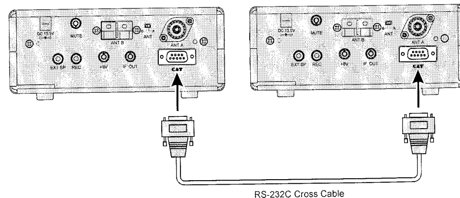
RS-232C Cross Cable
