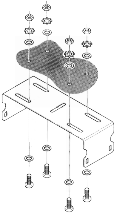
〔第3図〕MMB-33の取付け方法
