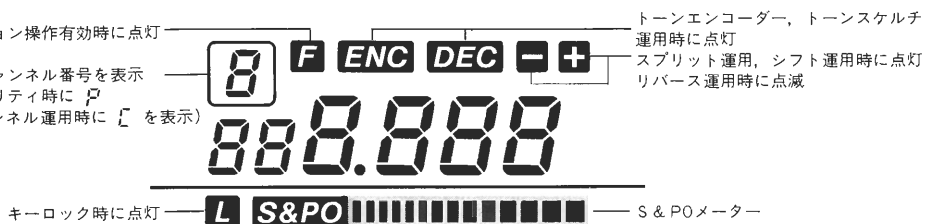
〔第1図〕ディスプレイ
