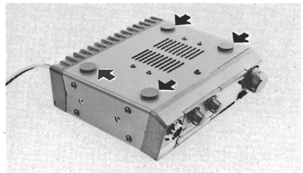
[写真3]ゴム足の取付け位置
