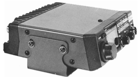
〔写真1〕固定運用時にもMMB-33
