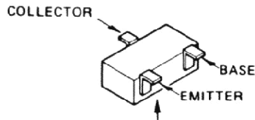
Marked Surface DTA143EK (3C) (Q1020, Q1022)
