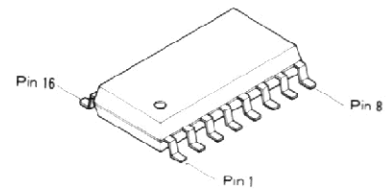
MC145158F2 (Q1024) MC3372M (Q1008)
