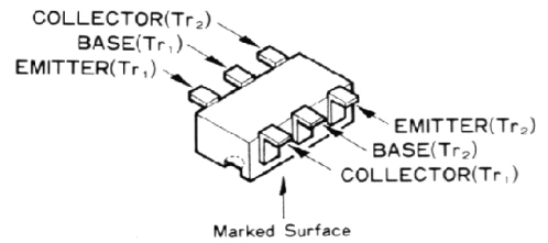
IMD2 (D2) (Q2006)
