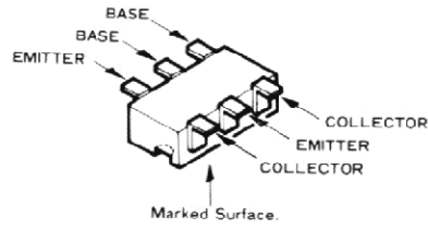
IMX3 (X3) (Q1026)
