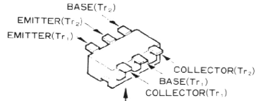
IMH5 (H5) (Q1006, Q1021)
