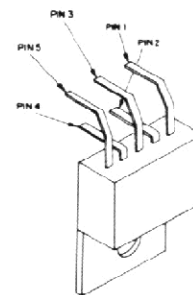
TDA2003H (Q1023)
