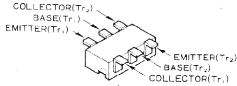
IMX3 (X3) (Q1026)
