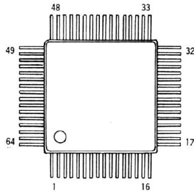
LC7582 (Q2002)
