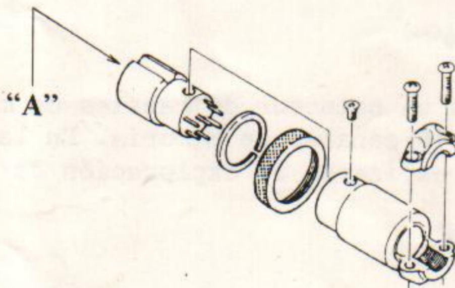
CONEXIONES DE MICROFONO
