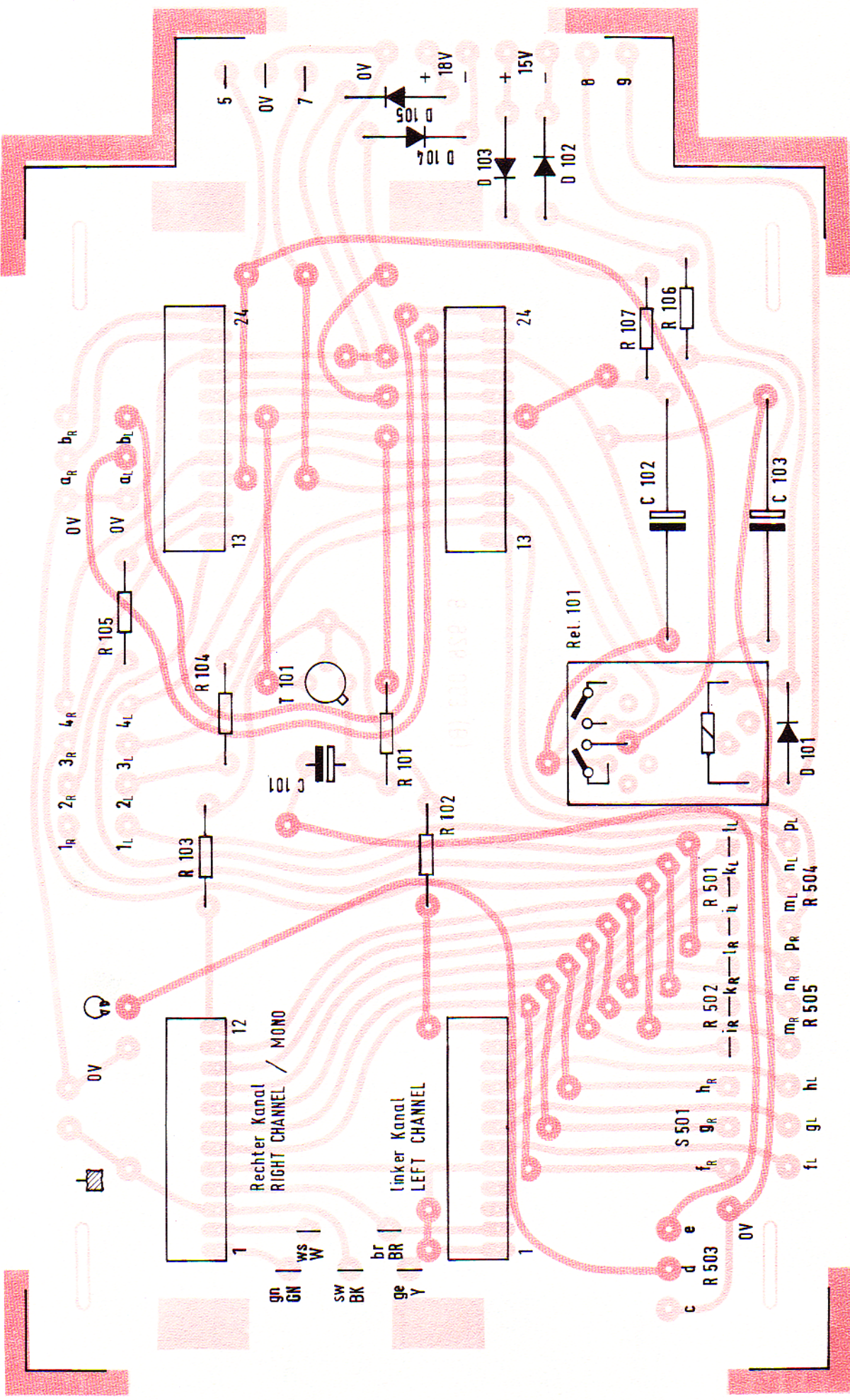
Grundplatte Verstärker Base board amplifier
