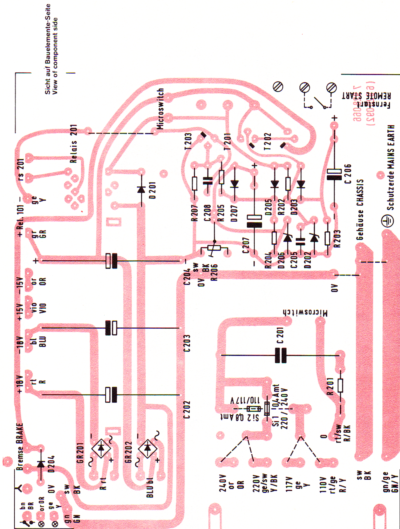
Netzteilplatte Power supply
