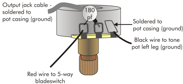
Volume pot wiring:
