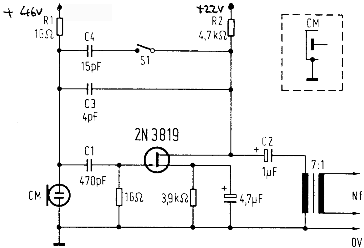
Grundschtung eines einstufigen Nf-Kondensator-Mikrofons
