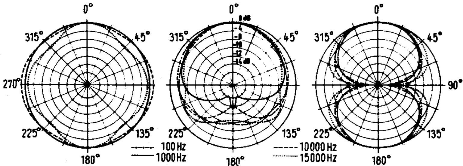
Bild E 21. Schaltung eines Mikrofons mit umschaltbarer Richtcharakteristik
