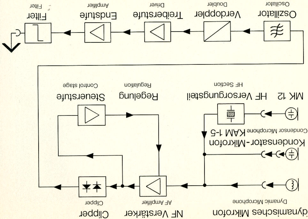
Bild 2 Blockschaubild des Taschensenders „SK 1007“
