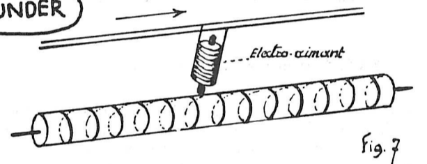
Fig. 7. — Principe d'un appareil Poulsen avec électro-aimant à mouvement transversal, et cylindre tournant portant le fil d'acier enroulé en hélice
