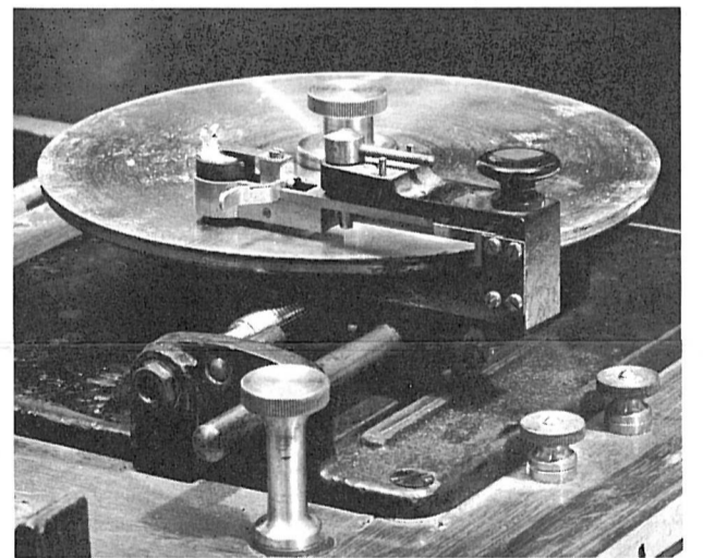
Fig. 7. — Principe d'un appareil Poulsen avec électro-aimant à mouvement transversal, et cylindre tournant portant le fil d'acier enroulé en hélice
