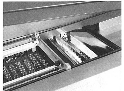
Chip-Bauteile kurz vor dem Zinnbad.
