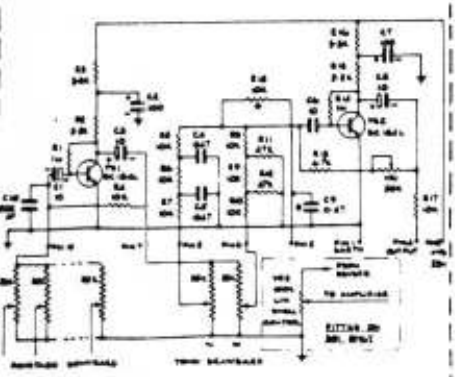
PRE-AMPLIFIER UNIT P.C.B. 104 02
