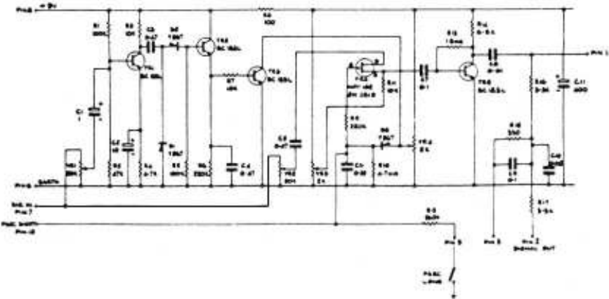
PRECISION UNIT P.C.B. 104 02
