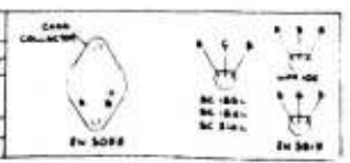
PRECISION UNIT P.C.B. 104 02
