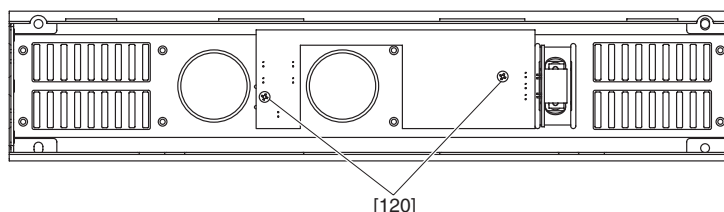
[90]: Bind Head Tapping Screw-S 3.0X6 MFZN2BL (EP630210)+バインドSタイト [120]: Bind Head Tapping Screw-S 3.0X6 MFZN2BL (EP630210)+バインドSタイト [360]: Hex Socket Tapping Screw-S3.0X10 MFZN2BL (WD345200)六角穴付きSタイト
